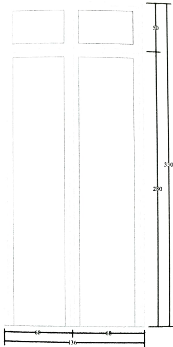
DETAIL PINTU 2
