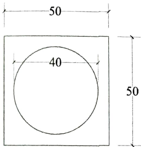
DETAIL KOLOM 2A 1 1 12
