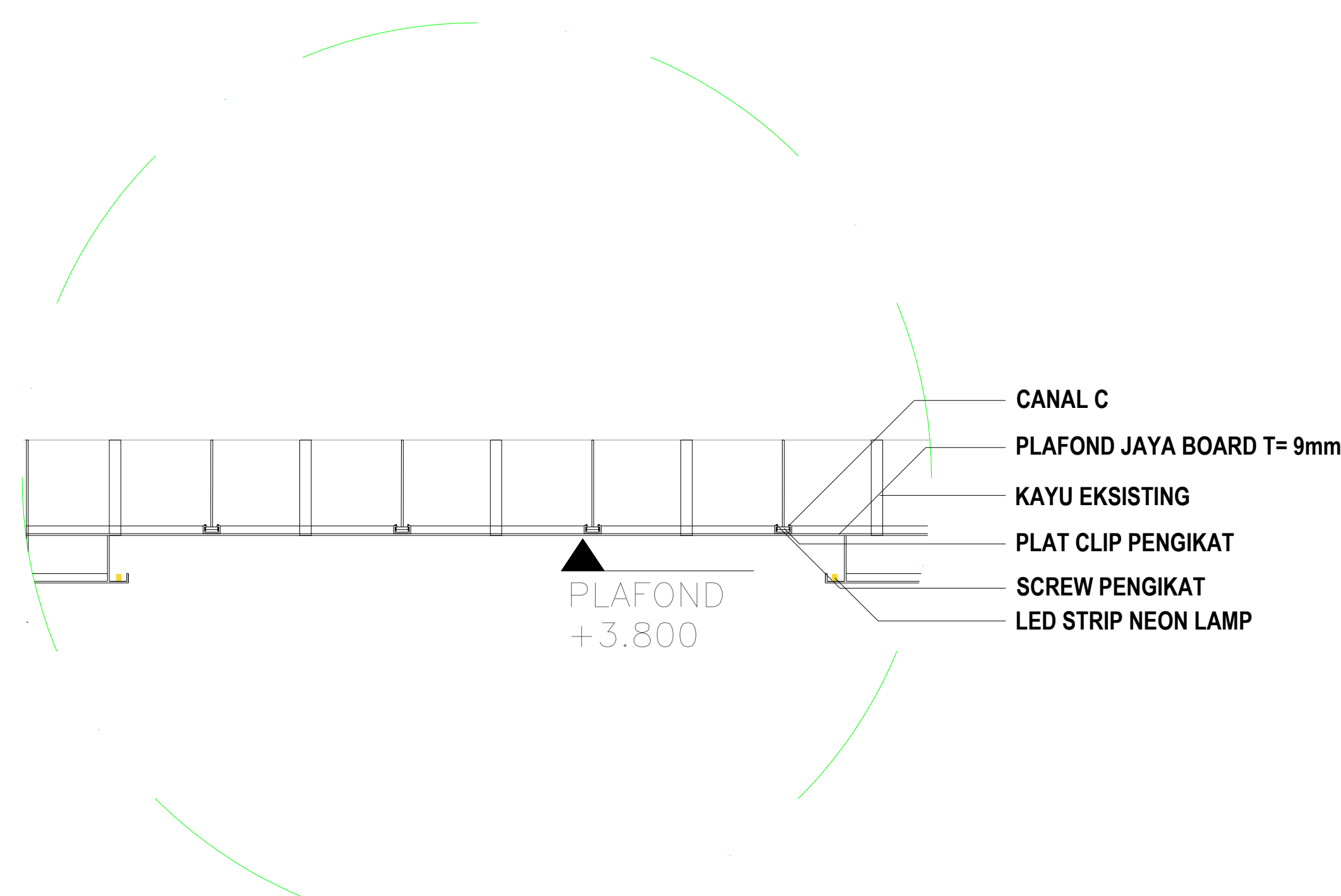
DETAIL PLAFOND Scale 1 : 50
