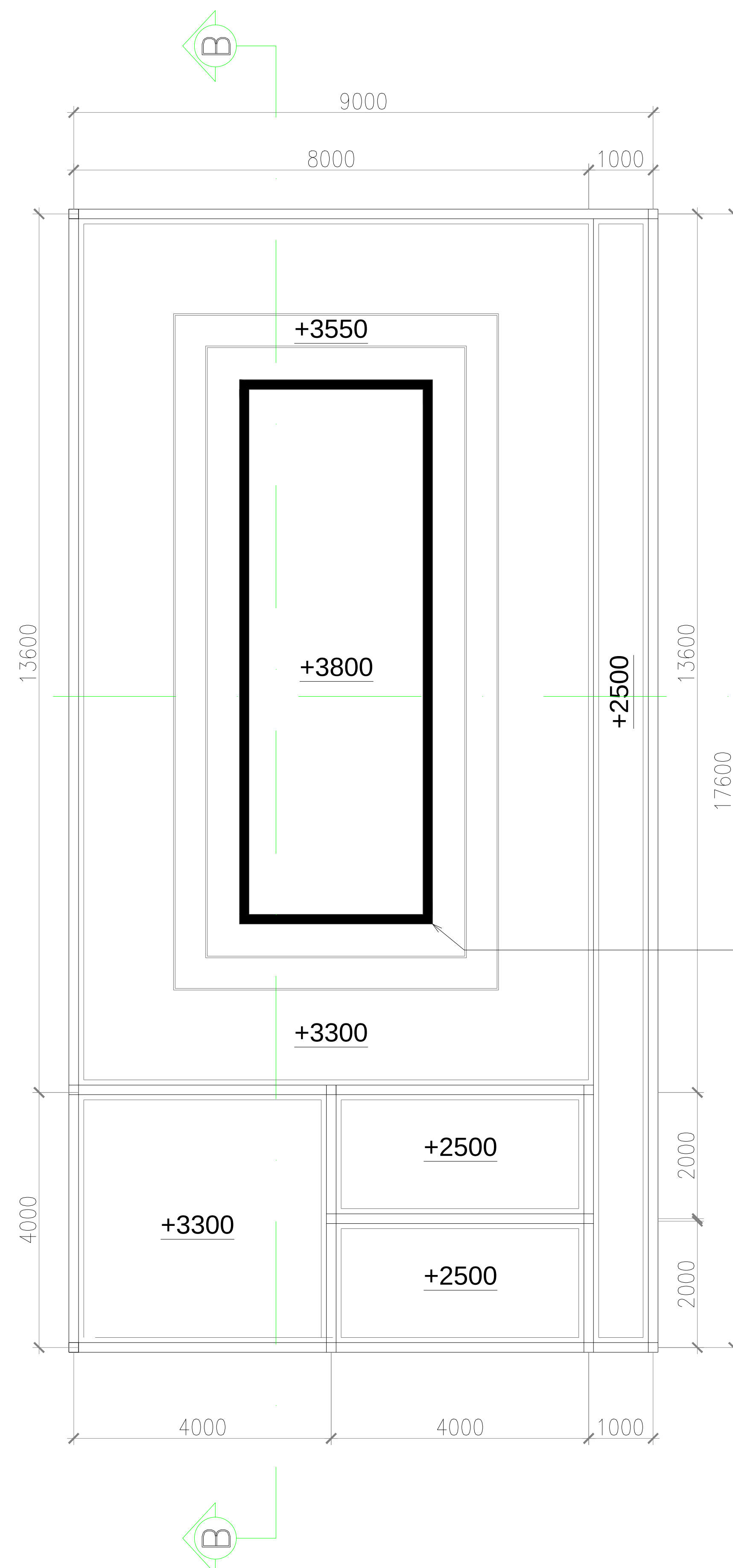
RENCANA PLAFOND LOBBY AULA Scale 1 : 100
