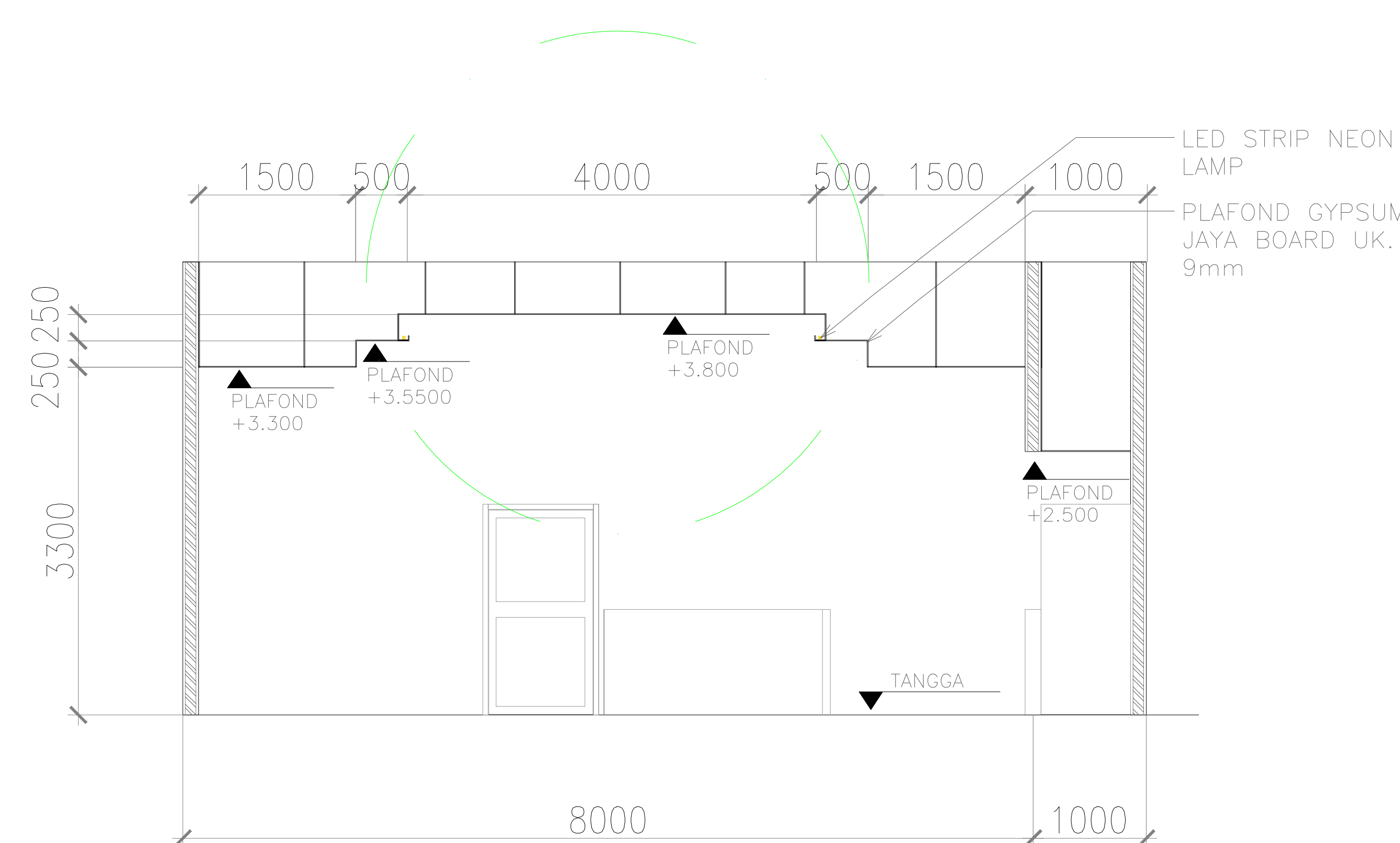
POTONGAN A-A LOBBY AULA Scale 1 : 75
