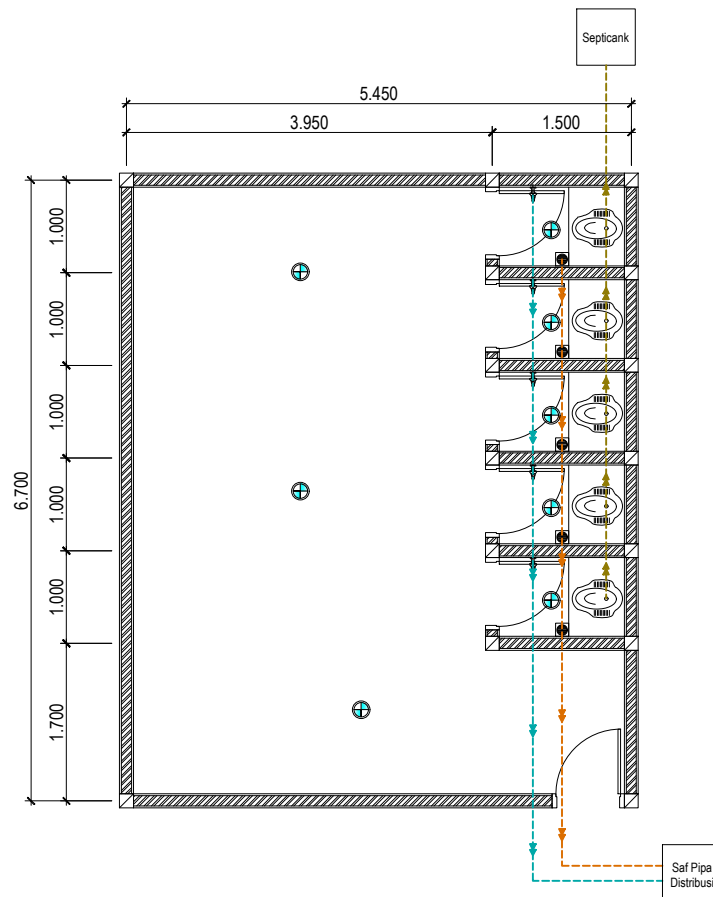
GSG ARS 1:75 DENAH INSTALASI MEKANIKAL & ELEKTRIKAL
