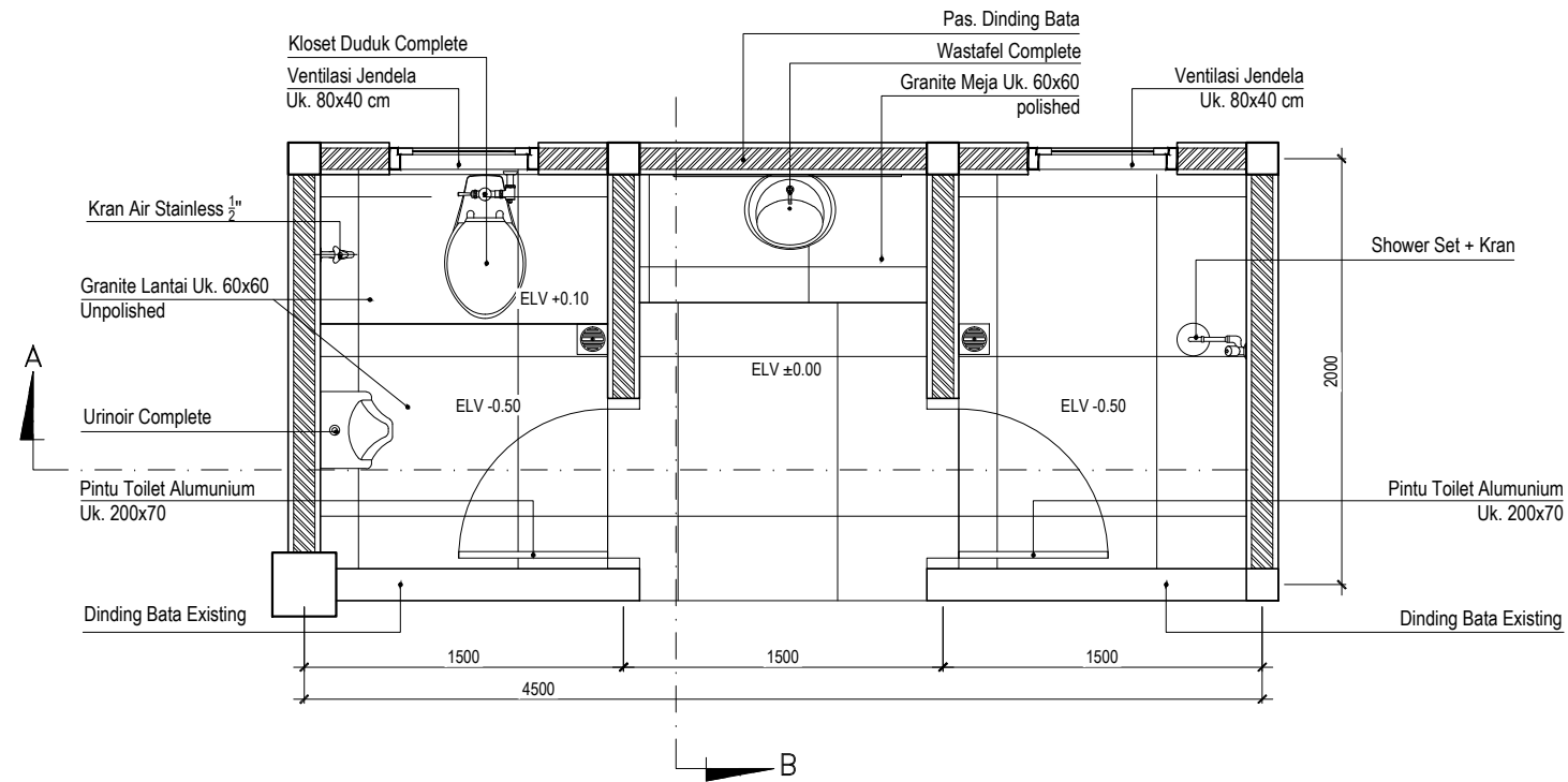
GSG ARS 1:35 DENAH TOILET VIP
