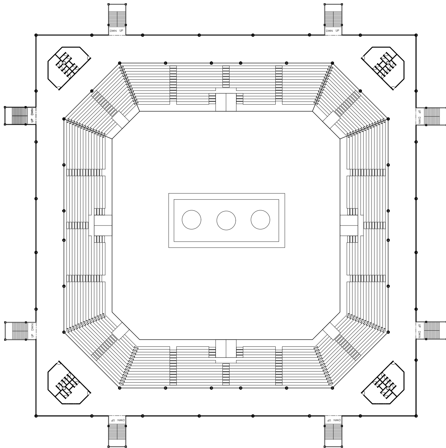
GSG ARS 1:500 DENAH GEDUNG SERBAGUNA LT.2
