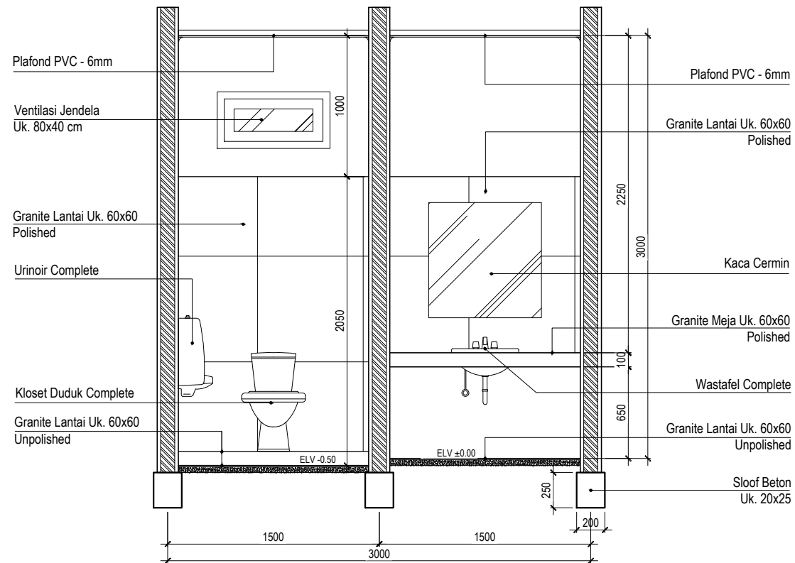
GSG ARS 1:35 DETAIL POTONGAN A-A
