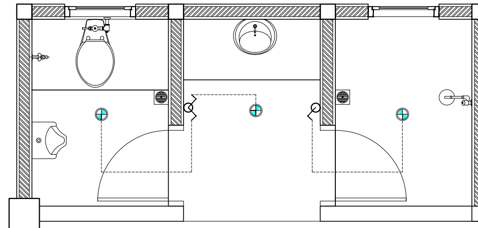
GSG ARS 1:35 DENAH INSTALASI ELEKTRIKAL
