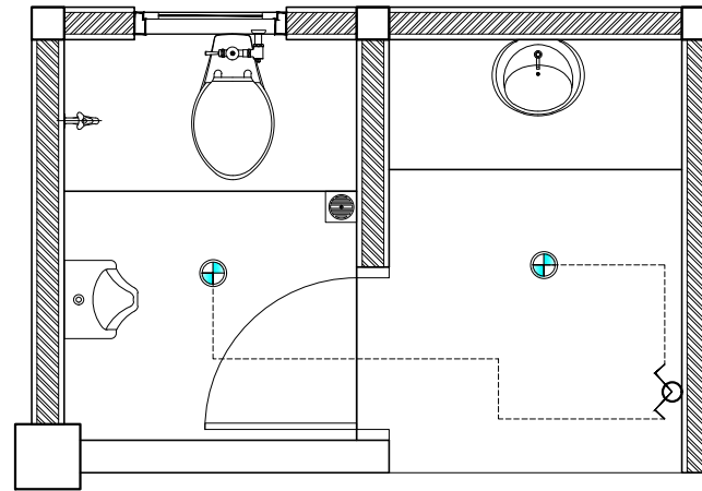
GSG ARS 1:35 DENAH INSTALASI ELEKTRIKAL
