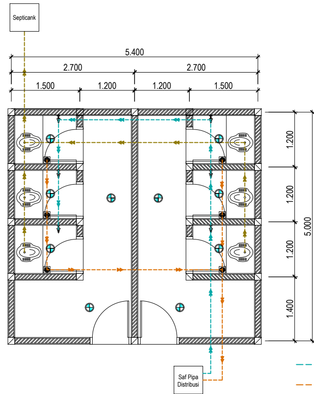
GSG ARS 1:75 DENAH INSTALASI MEKANIKAL & ELEKTRIKAL
