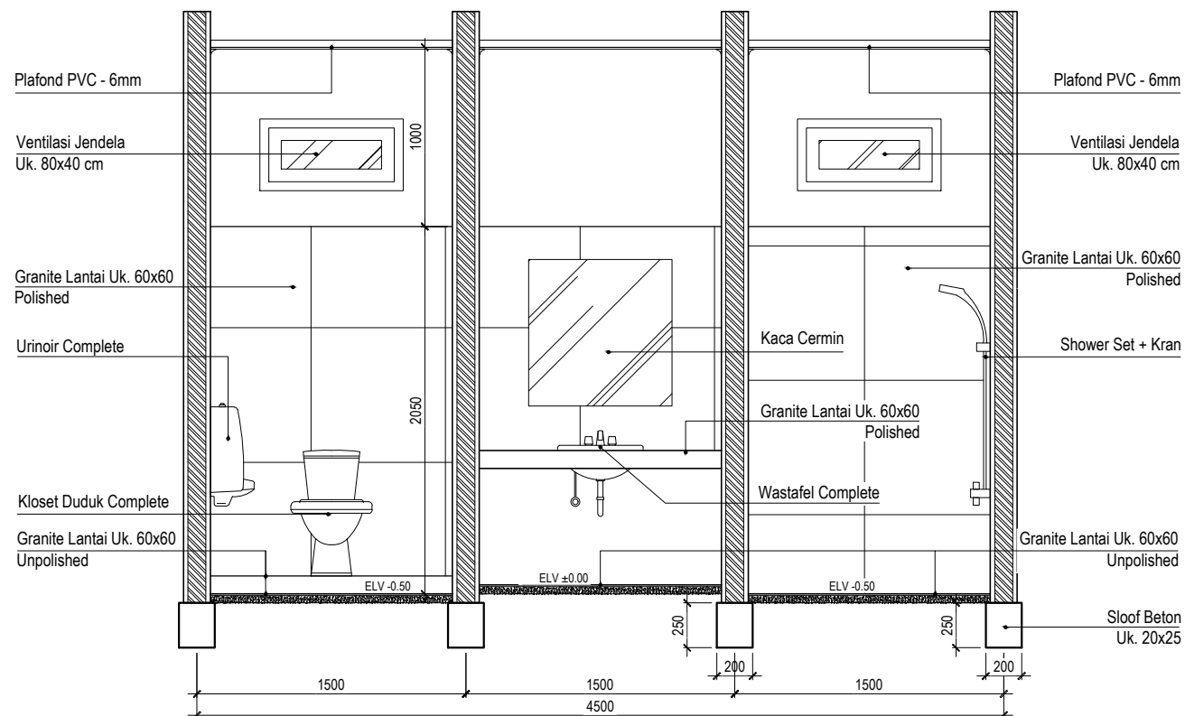
GSG ARS 1:35 DETAIL POTONGAN A-A
