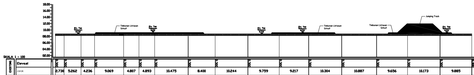
POTONGAN MELINTANG STA 0 + 140
