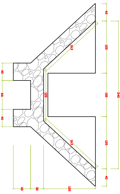
POTONGAN RENCANA BOX BSF4
