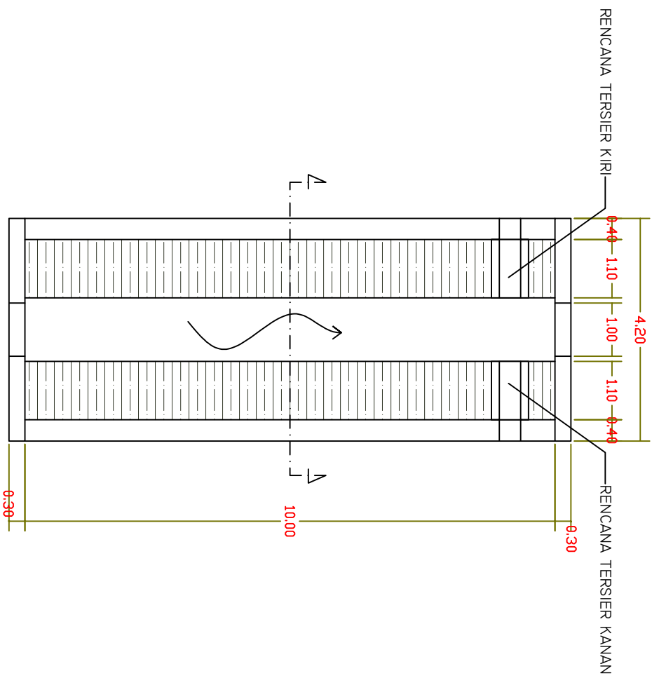
DENAH RENCANA BOX BSF4
