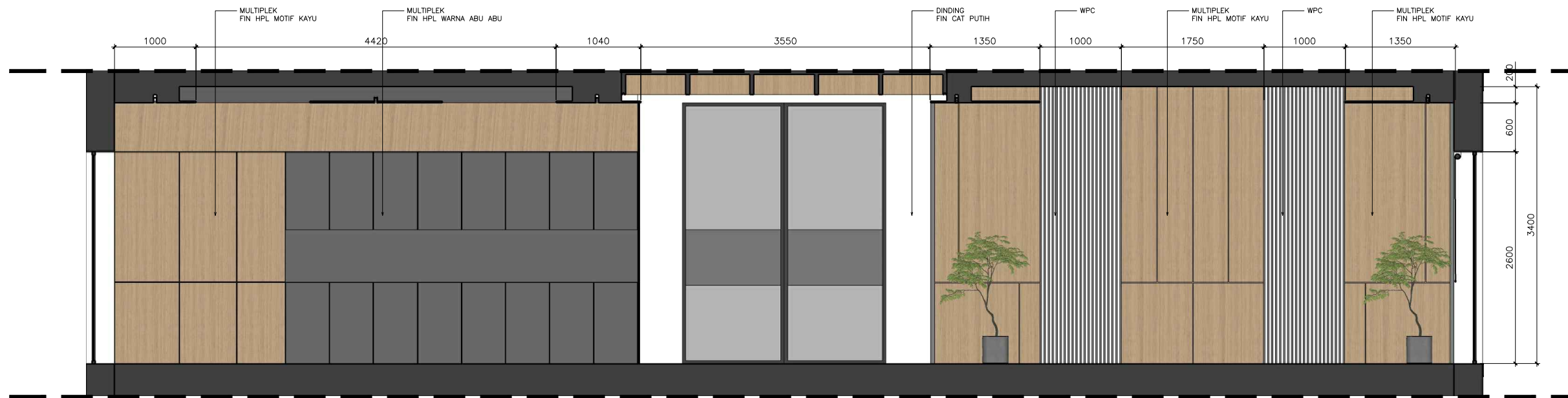
POTONGAN II 1 : 60
