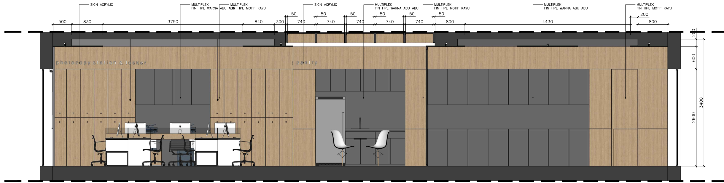
POTONGAN HH 1 : 60
