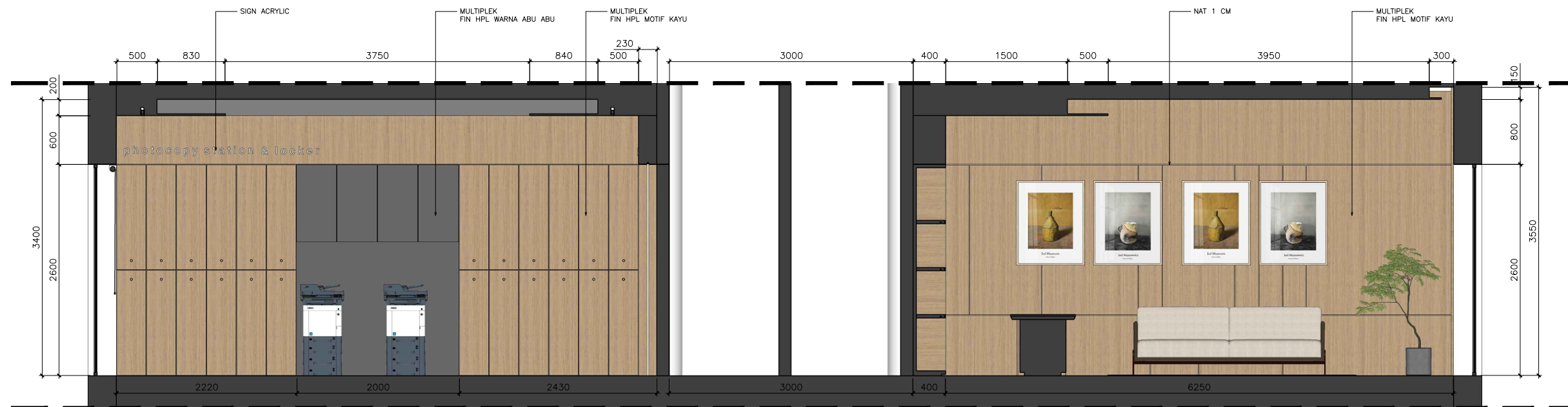
POTONGAN FF 1 : 60
