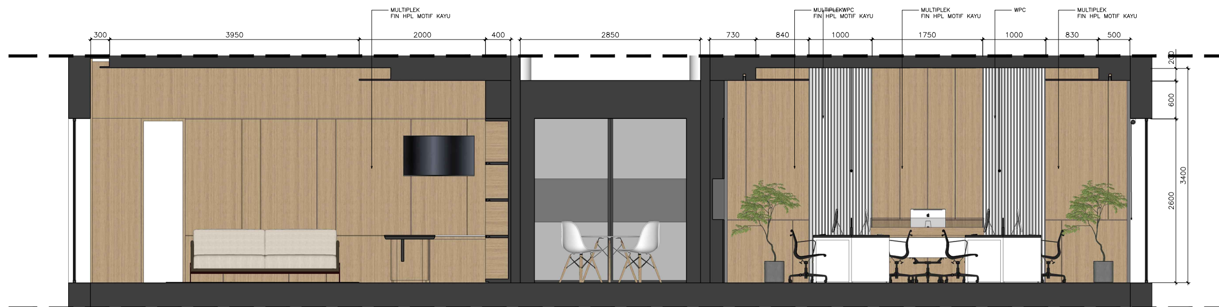
POTONGAN GG 1 : 60
