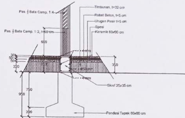
POT 2 Rg. Apotek SKALA 1 : 30
