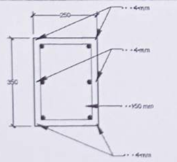
POT 1 Poli TB Dots SKALA 1 : 10
