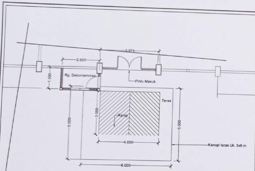
DENAH Entrance Pintu Masuk Gedung B SKALA 1 : 100
