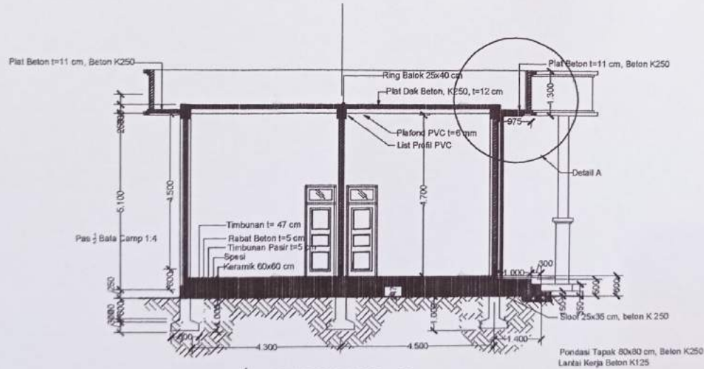
POTONGAN B - B Poli TB Dots SKALA 1 : 100
