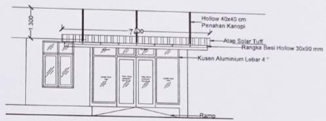
TAMPAK DEPAN Entrance Pintu Masuk Gedung B SKALA 1 : 100
