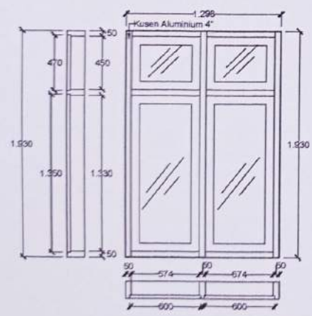
KUSEN J2 (2 UNIT) GEDUNG GIZI SKALA 1 : 30
