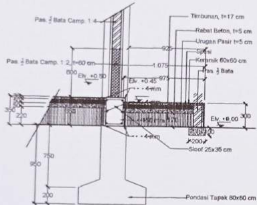
POT 1 Rg. Apotek SKALA 1 : 30
