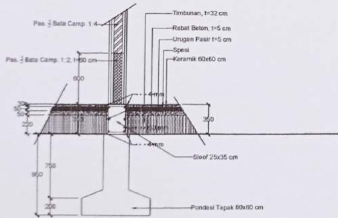
POT 3 Rg. Apotek SKALA 1 : 30
