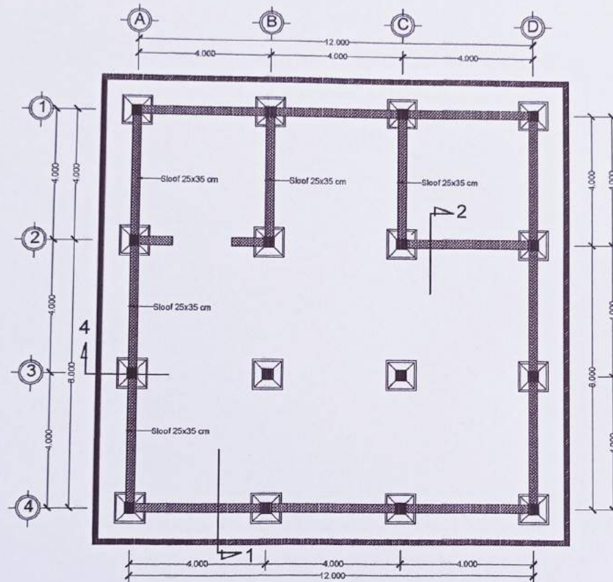
RENCANA PONDASI DAN SLOOF GEDUNG GIZI SKALA 1 : 100
