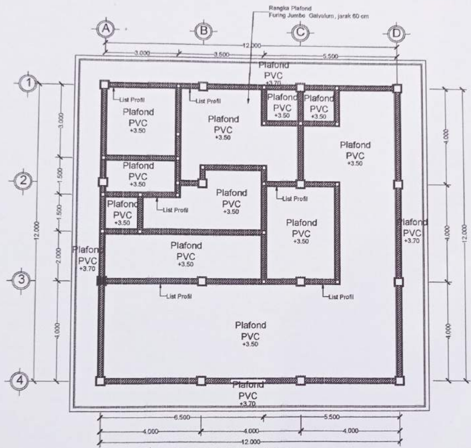
RENCANA PLAFOND Rg. Apotek SKALA 1 : 100
