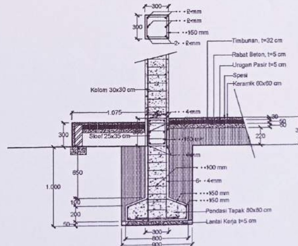
POTONGAN 4 GEDUNG GIZI SKALA 1 : 30
