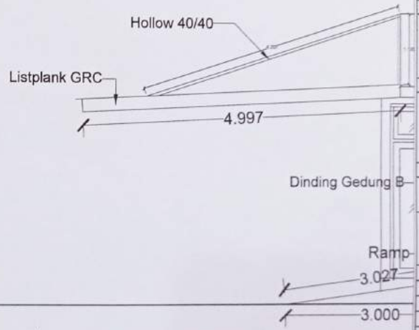
TAMPAK SAMPIING Entrance Pintu Masuk Gedung B SKALA 1 : 100
