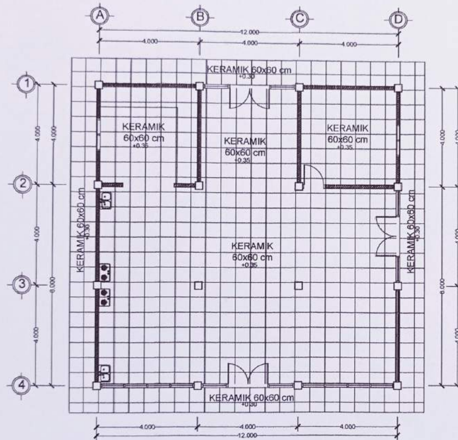
RENCANA KERAMIK LANTAI GEDUNG GIZI SKALA 1 : 100
