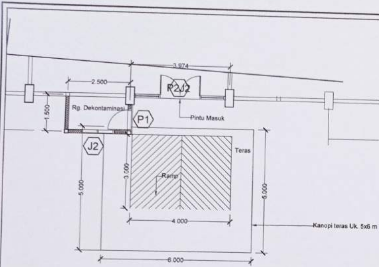
RENCANA KUSEN Entrance Pintu Masuk Gedung B SKALA 1 : 100
