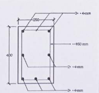
POT 3 Poli TB Dots SKALA 1 : 10
