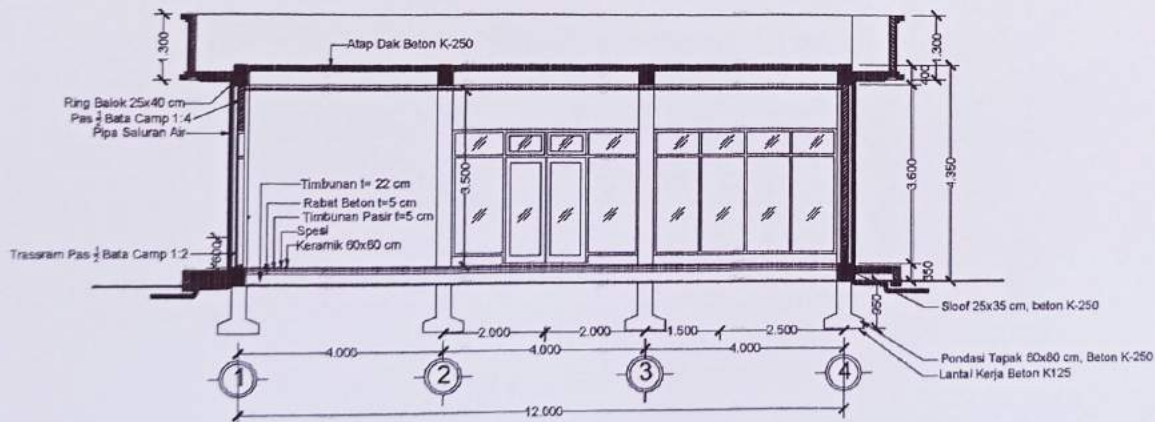
POTONGAN B - B GEDUNG GIZI SKALA 1 : 100
