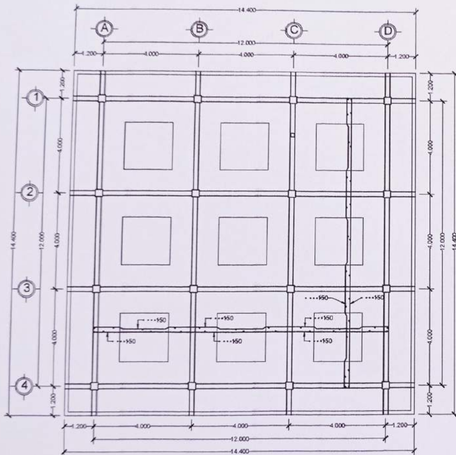
RENCANA PEMBESIAN PLAT LANTAI GEDUNG GIZI SKALA 1 : 100
