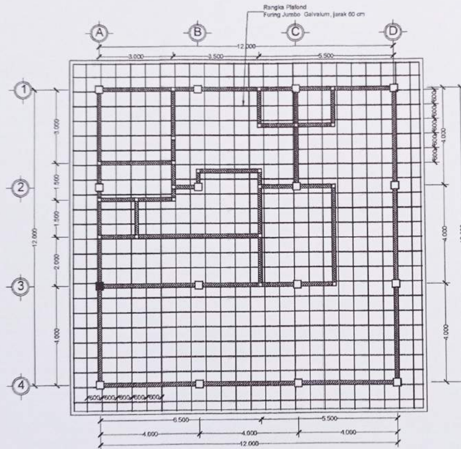
RENCANA RANGKA PLAFOND Ry. Apriok SKALA 1 : 100
