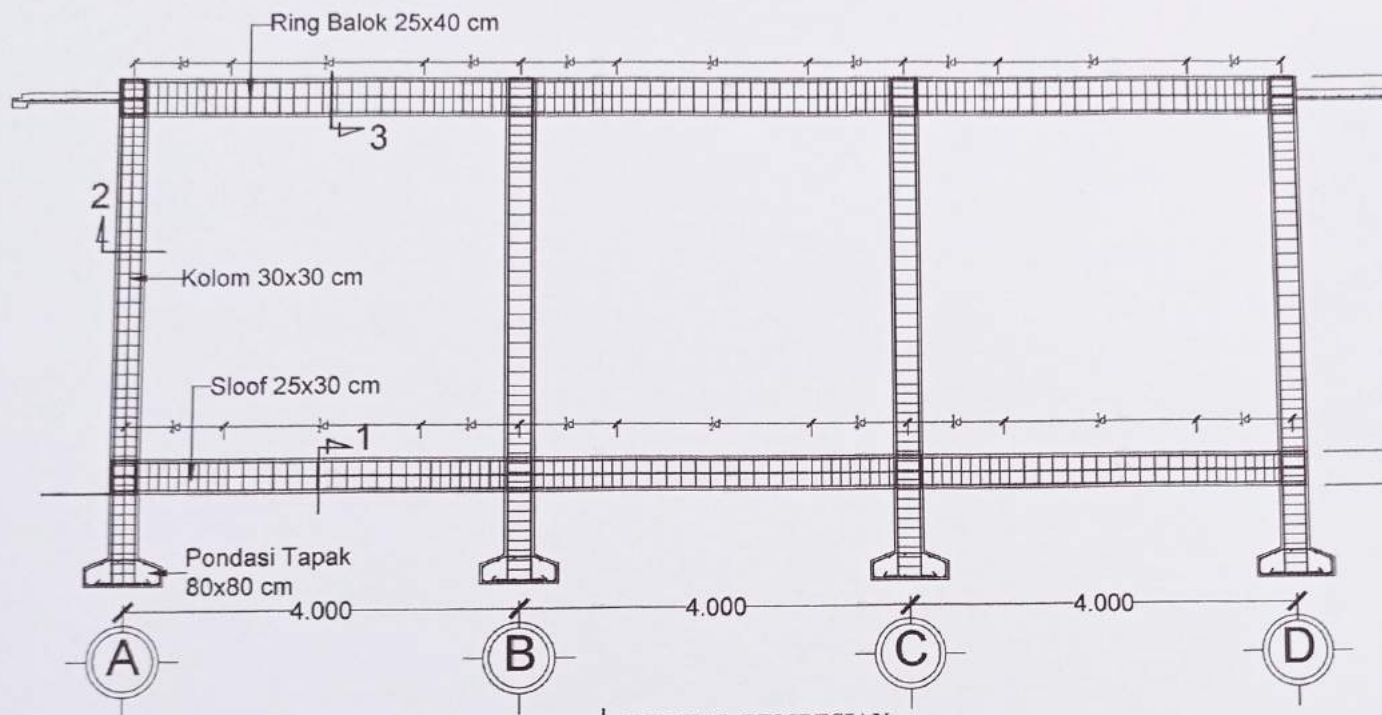
PORTAL PEMBESIAN Rg. Apotek SKALA 1 : 50
