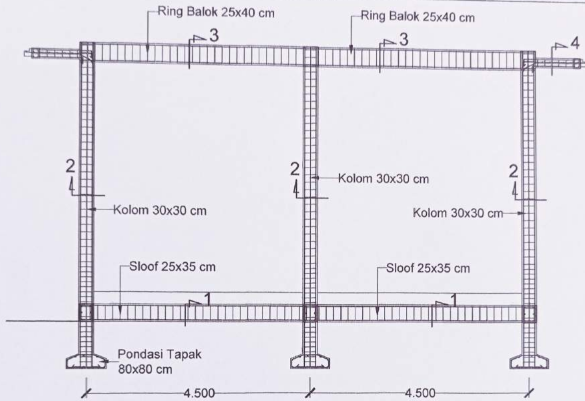
PORTAL PEMESIAN Poli TB Dots SKALA 1 : 50
