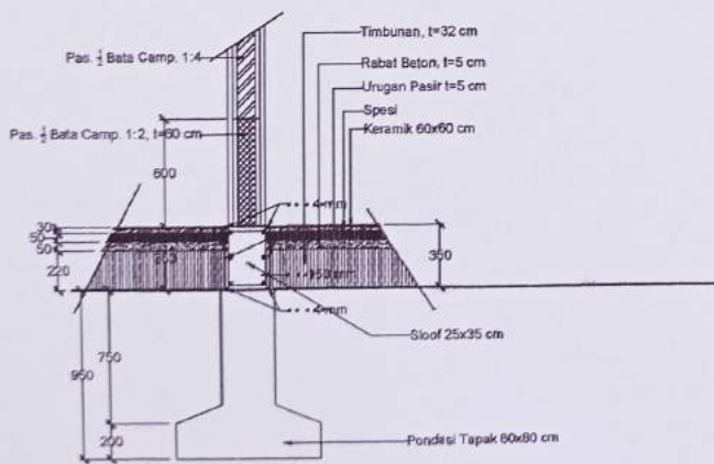
POTONGAN 2 GEDUNG GIZI SKALA 1 : 30
