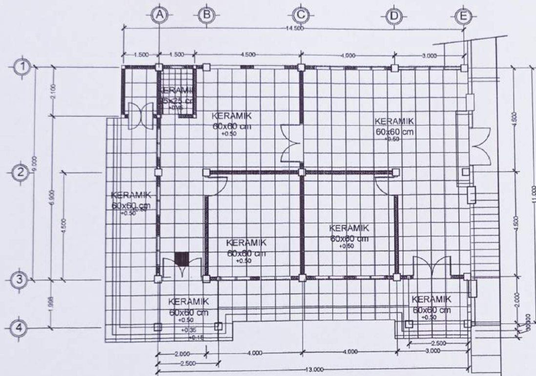
RENCANA LANTAI KERAMIK Pol: TB Dots SKALA 1 : 100
