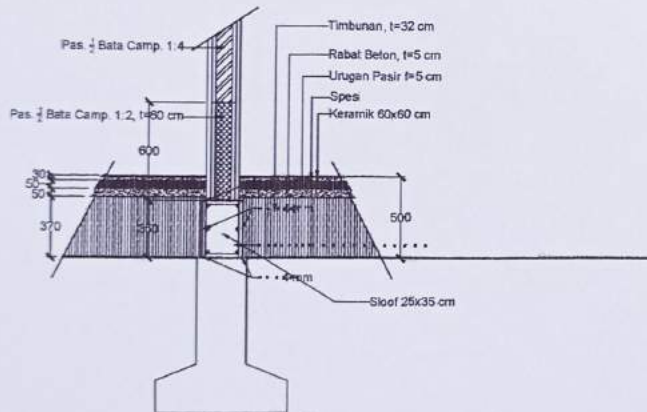
POTONGAN 3 Poli TB Dots SKALA 1 : 30
