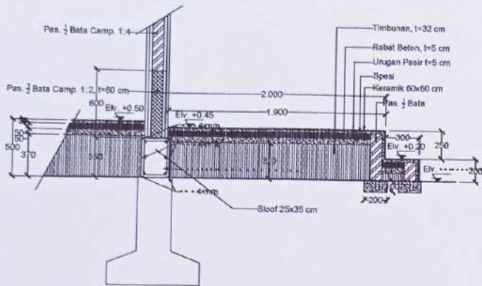
POTONGAN 1 Poli TB Dots SKALA 1 : 30
