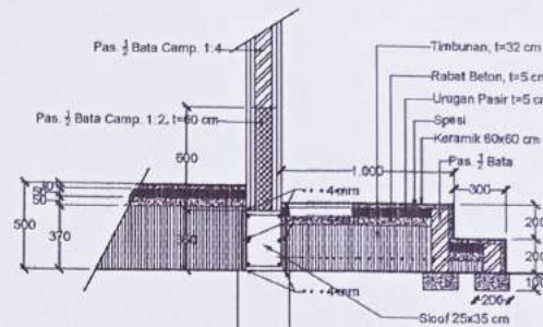
POTONGAN 2 Poli TB Dots SKALA 1 : 30
