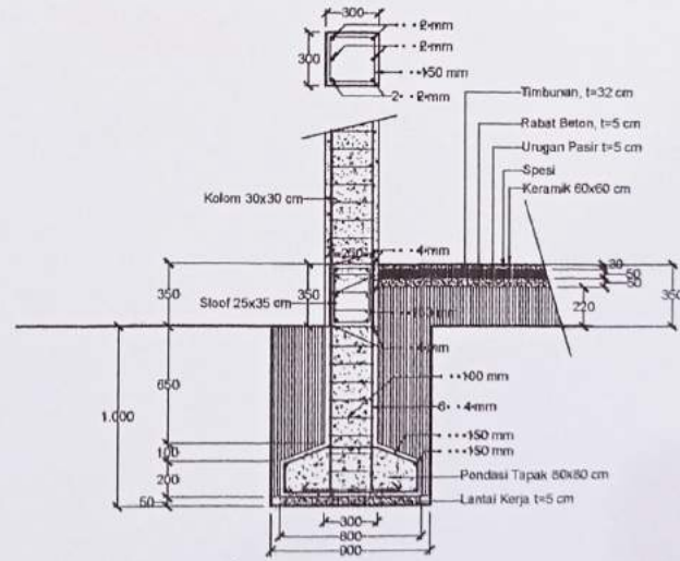
POT. 4 Rg. Apotek SKALA 1 : 30
