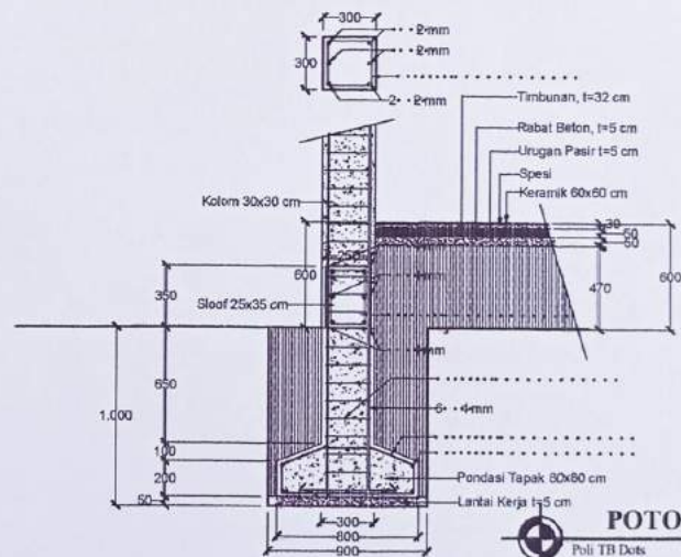
POTONGAN 2 Poli TB Dots SKALA 1 : 30
