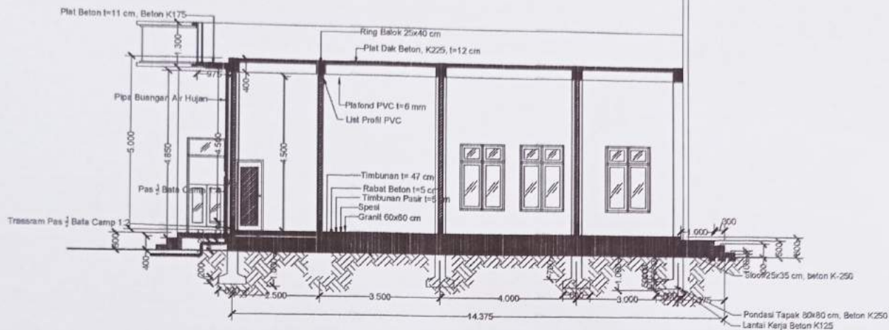
POTONGAN A - A Poli TB Dots SKALA 1 : 100
