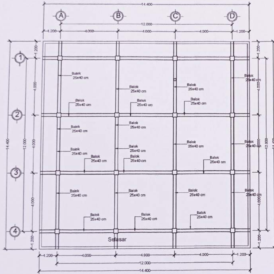
RENCANA BALOK GEDUNG GIZI SKALA 1 : 100
