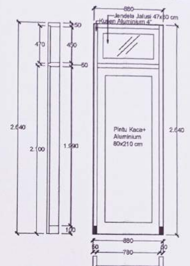
KUSEN P1 (1 UNIT) GEDUNG GIZI SKALA 1 : 30
