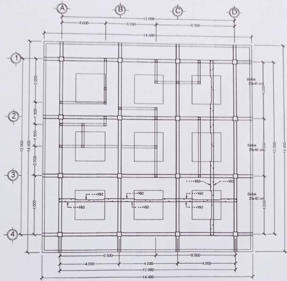
RENCANA PEMBESIAN PLAT LANTAI Rg. Aporek SKALA 1 : 100
