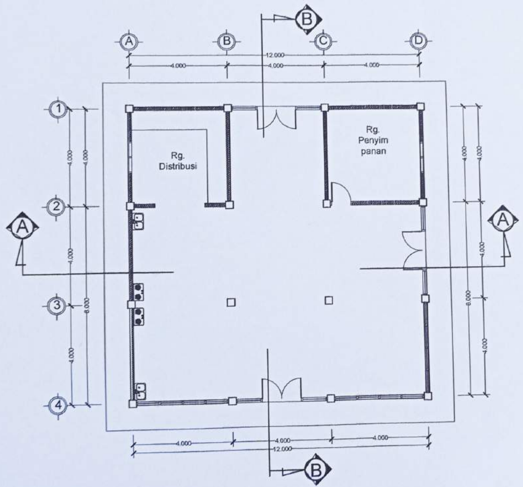
DENAH GEDUNG GIZI SKALA 1 : 100
