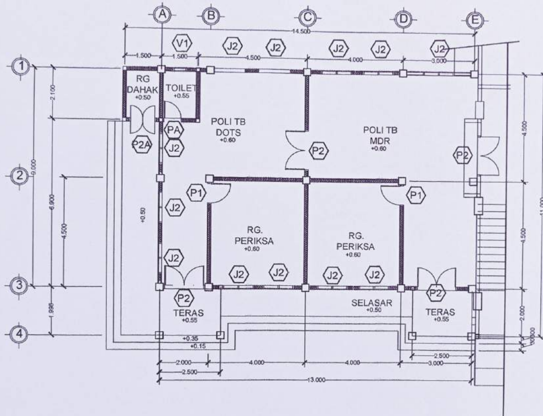
RENCANA KUSEN PINTU DAN JENDELA Polio TB Dots SKALA 1 : 100
