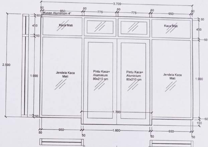
KUSEN P2J2 (1 UNIT) Entrance Pintu Masuk Gedung B SKALA 1 : 30
