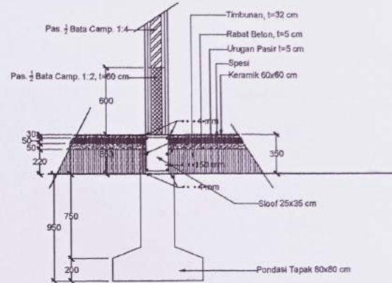
POTONGAN 3 GEDUNG GIZI SKALA 1 : 30
