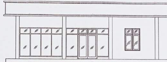
TAMPAK SAMPIING KANAN GEDUNG GIZI SKALA 1 : 100
