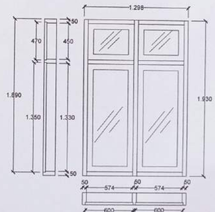
KUSEN J2 (1 UNIT) Entrance Pintu Masuk Gedung B SKALA 1 : 30
