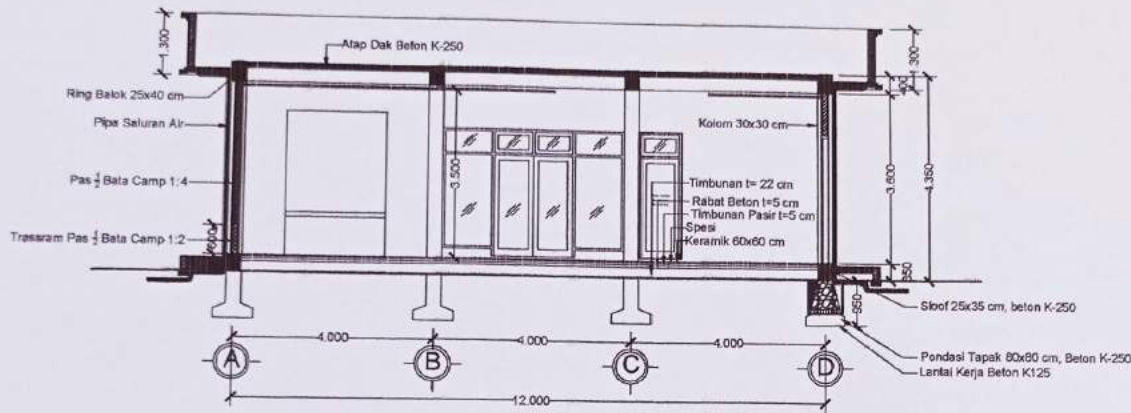
POTONGAN A - A GEDUNG GIZI SKALA 1 : 100
