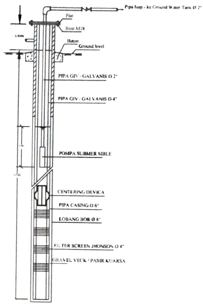
Detail Sumur Bor 1:25
