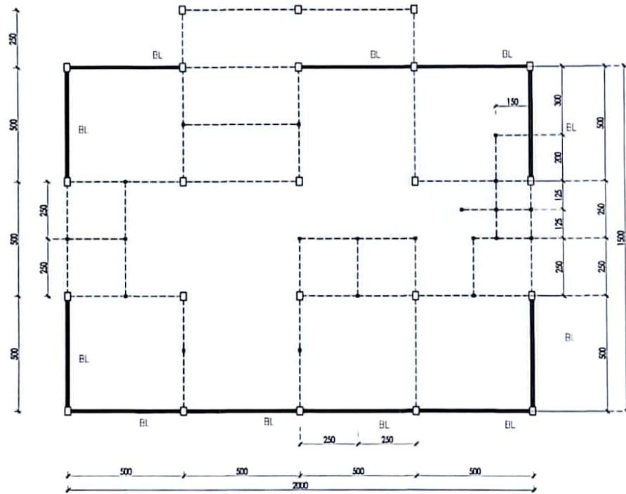
DENAH RENCANA BALOK LANTAI ELV. +2.29 SKALA 1:150
