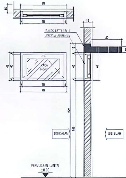
DETAIL VENTILASI V1 = 6 UNIT SKALA 1:20
