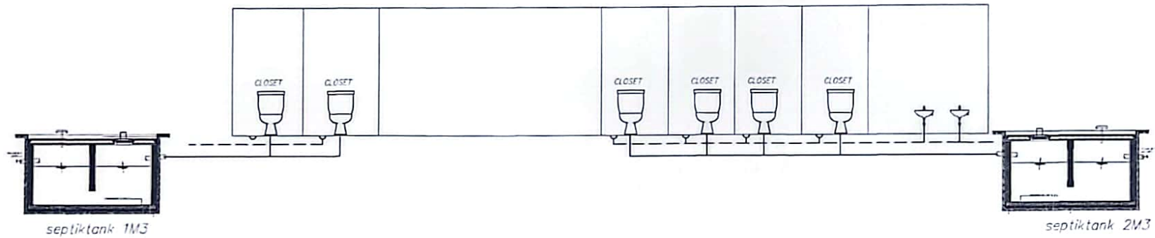
DIAGRAM INSTALASI PIPA AIR BEKAS DAN KOTOR SKALA 1:15
