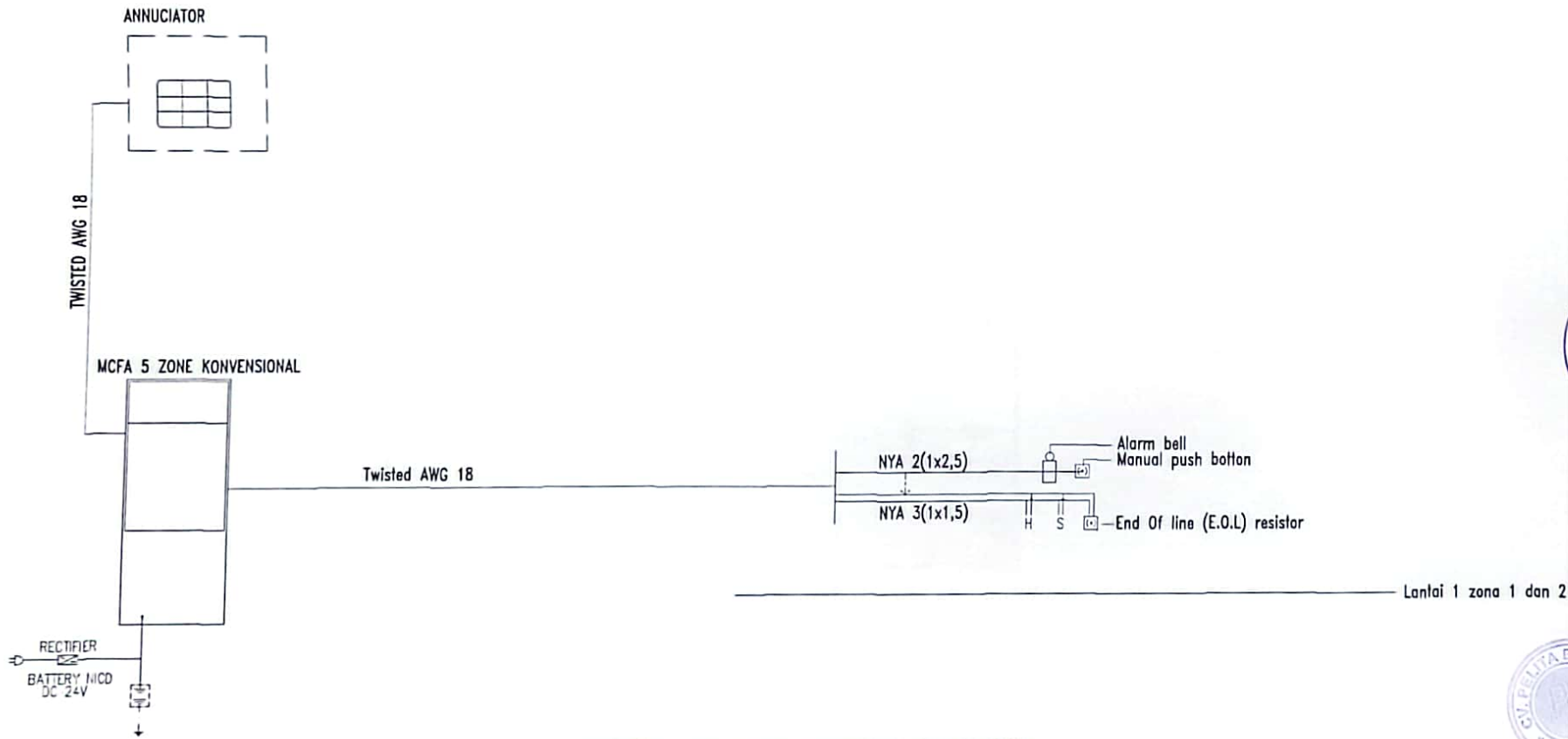
DIAGRAM SKEMATIK FIRE ALARM SKALA NTS
