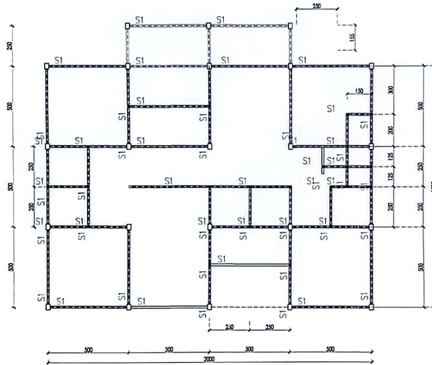
DENAH RENCANA SLOOF SKALA 1:150
