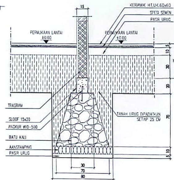
DETAIL 2 - 2 PONDASI MENERUS SKALA 1:20
