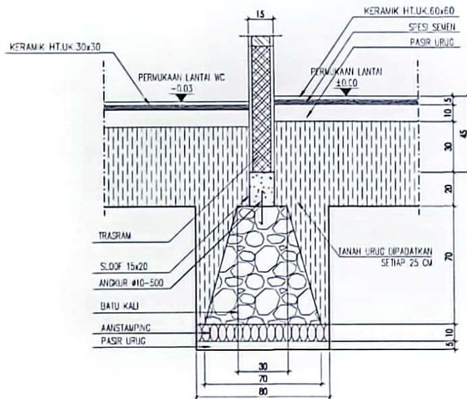
DETAIL 4-4 PONDASI MENERUS SKALA 1:20
