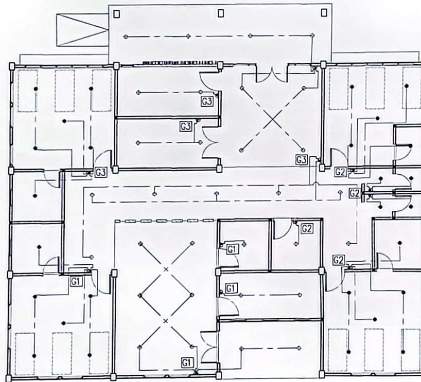
RENCANA TITIK LAMPU SKALA NTS
