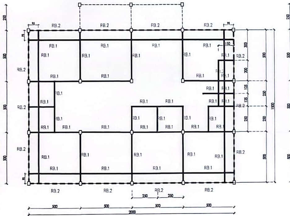
DENAH RENCANA RING BALOK ELV. +3.50 SKALA 1:150
