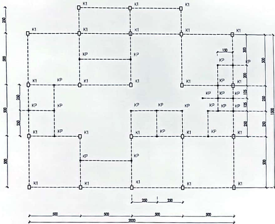
DENAH RENCANA KOLOM BAWAH SKALA 1:150
