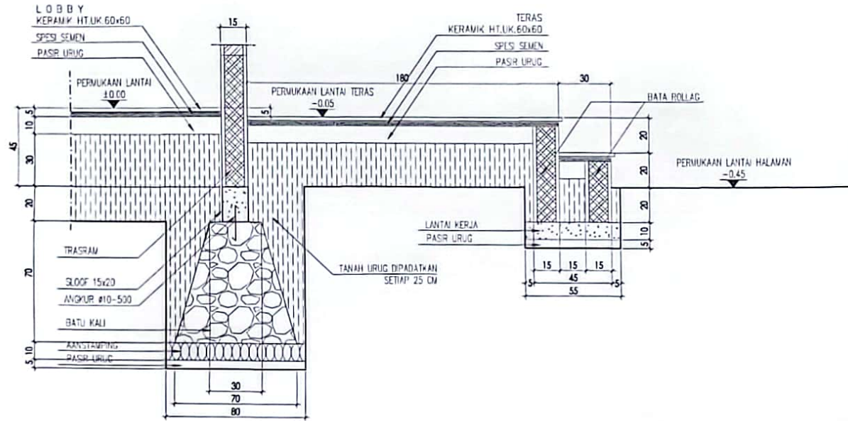
DETAIL 1 - 1 PONDASI MENERUS SKALA 1:20
