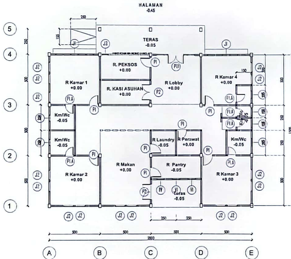
DENAH RENCANA KUSEN SKALA 1 : 150
