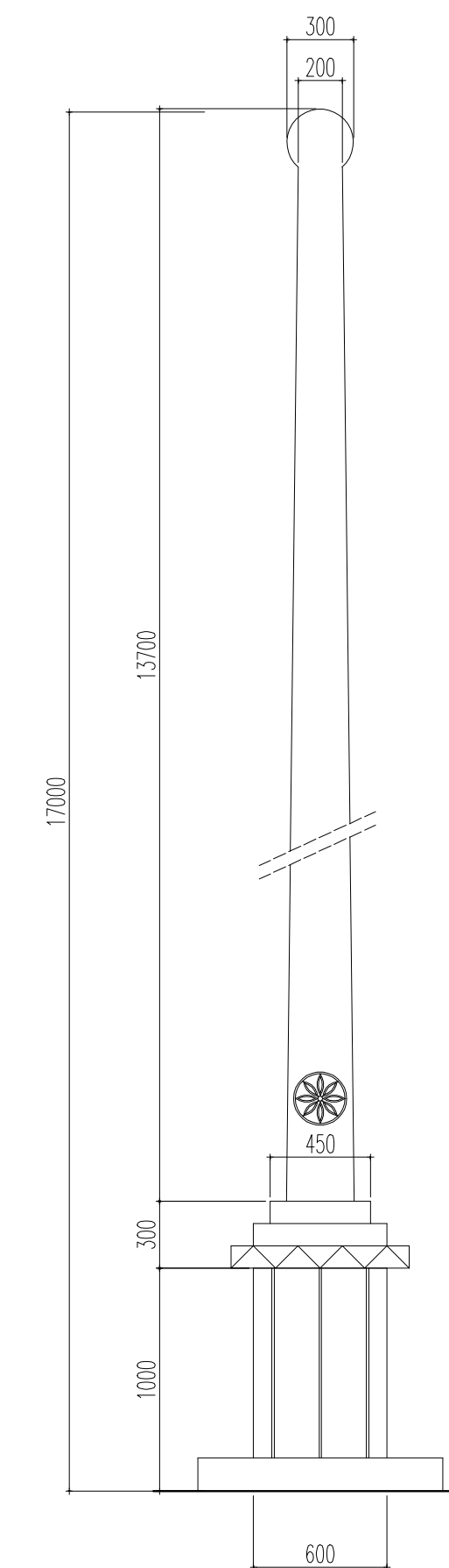
TAMPAK TIANG BENDERA SKALA 1:100
