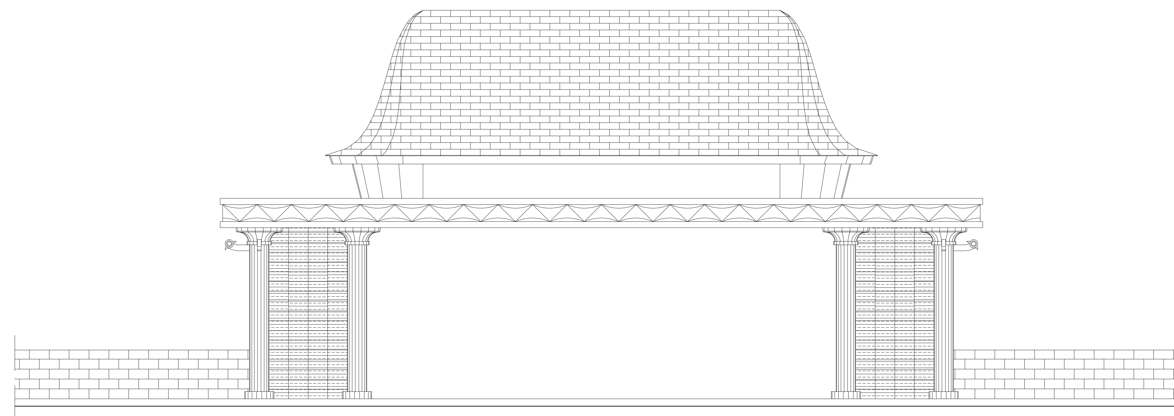
TAMPAK BELAKANG GAPURA SKALA 1:100
