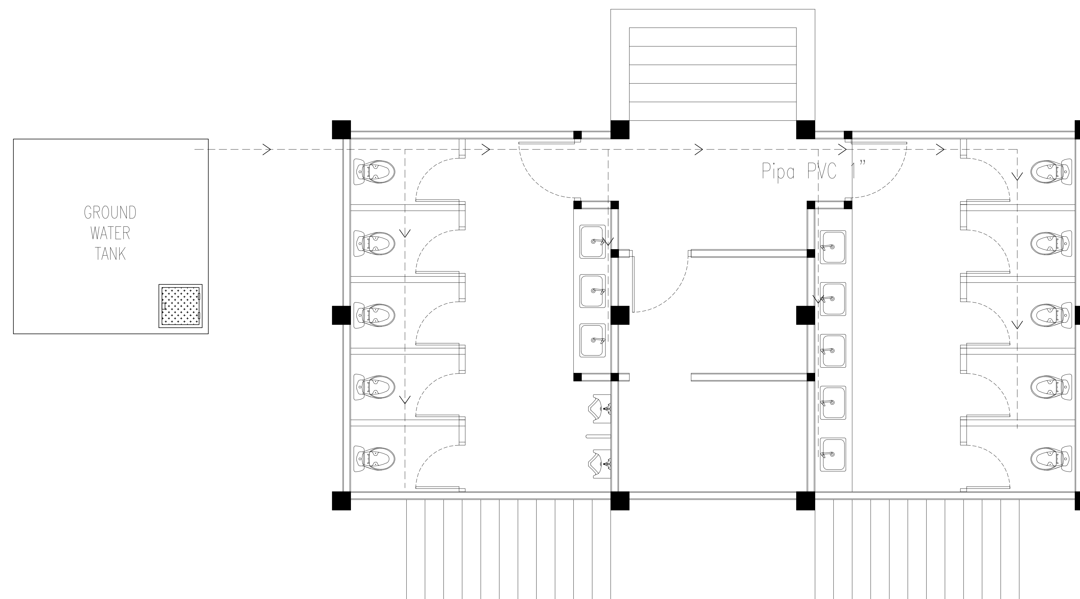
DENAH INSTALASI AIR BERSIH KAMAR MANDI SKALA 1:100
