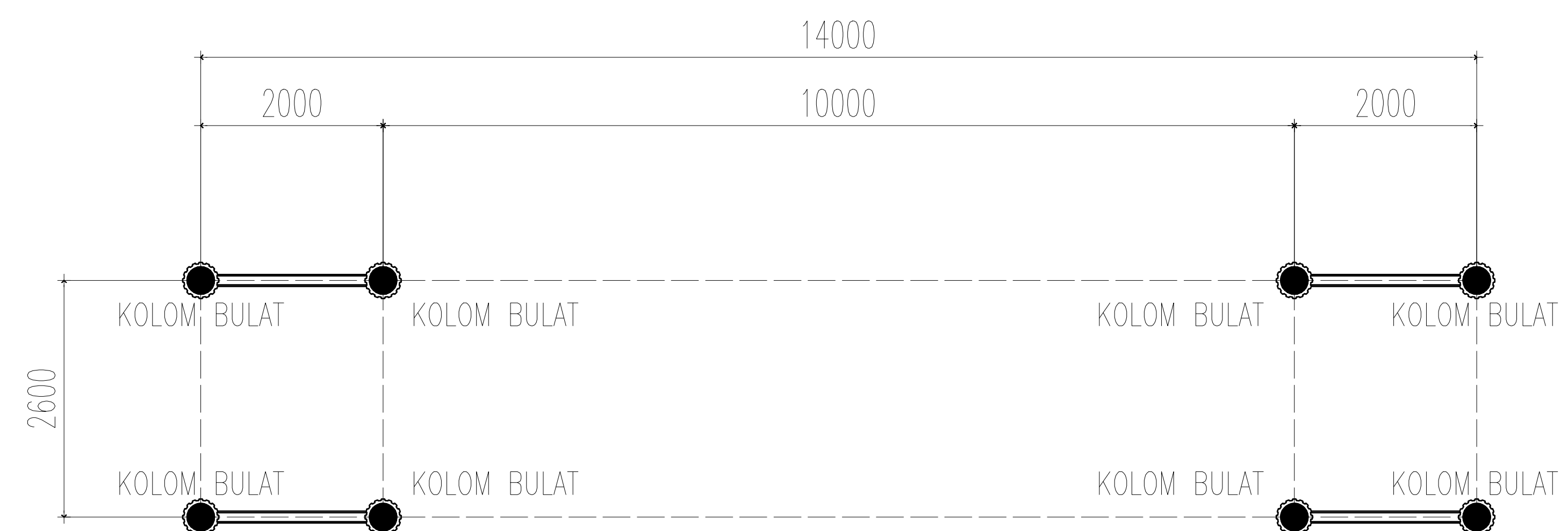
DENAH KOLOM SKALA 1:100
