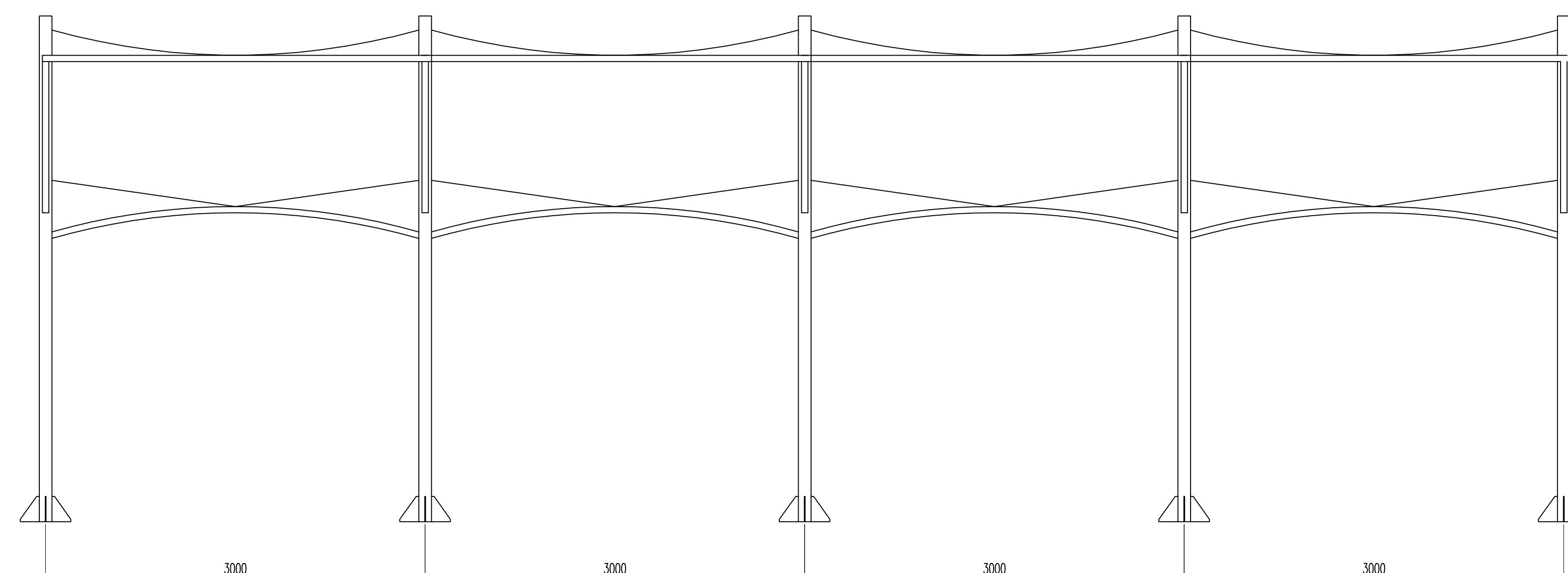
TAMPAK DEPAN ATAP KANOPI TRIBUN SKALA 1:100
