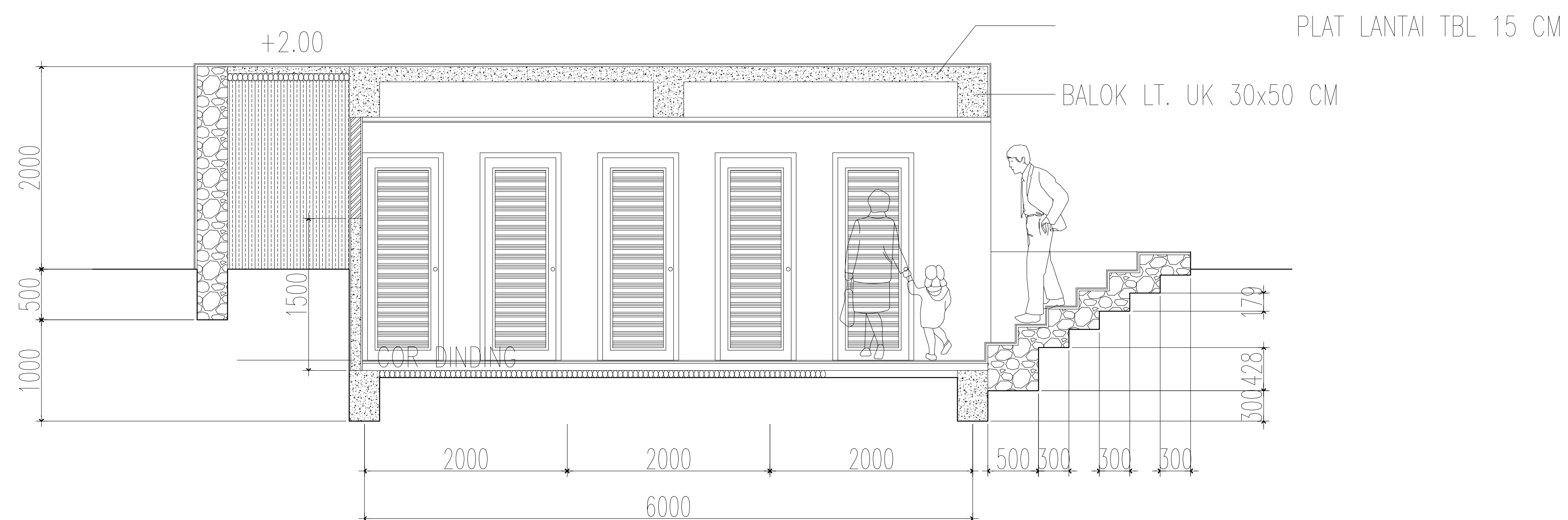
POTONGAN MELINTANG II SKALA 1:100
