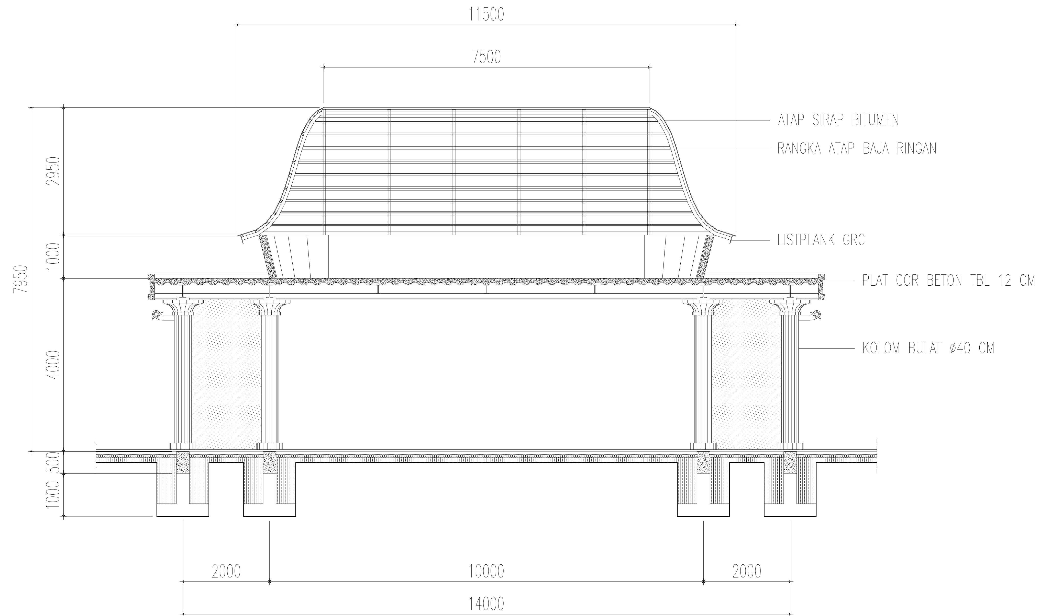
POTONGAN MELINTANG GAPURA SKALA 1:100
