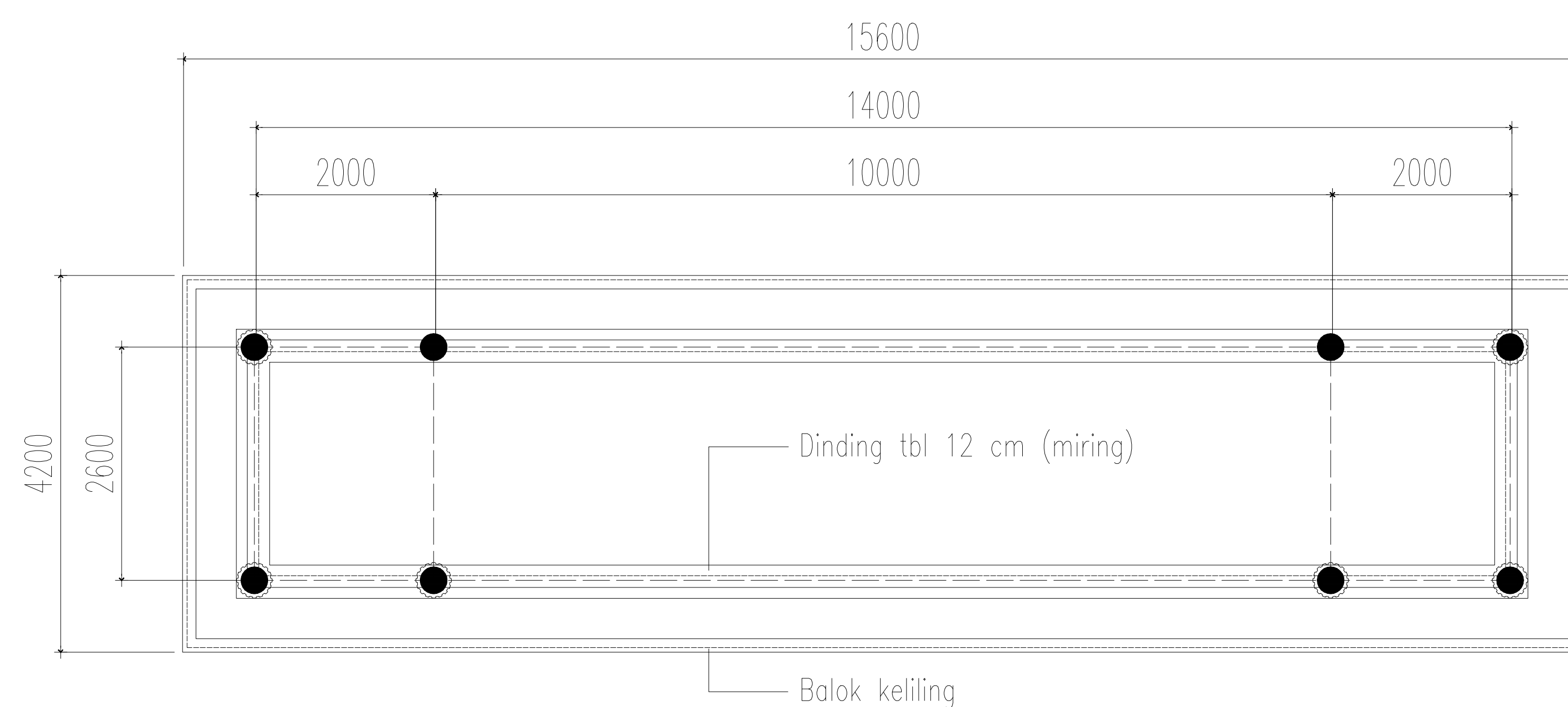
DENAH PLAT LANTAI BAWAH ATAP SKALA 1:100
