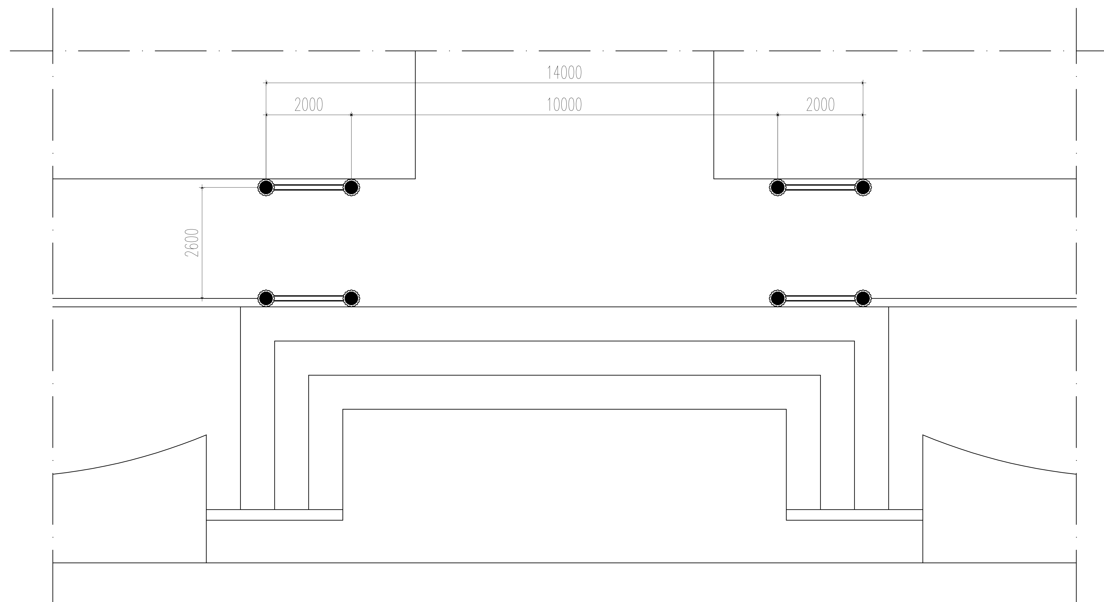
DENAH GAPURA LAPANGAN SKALA 1:100
