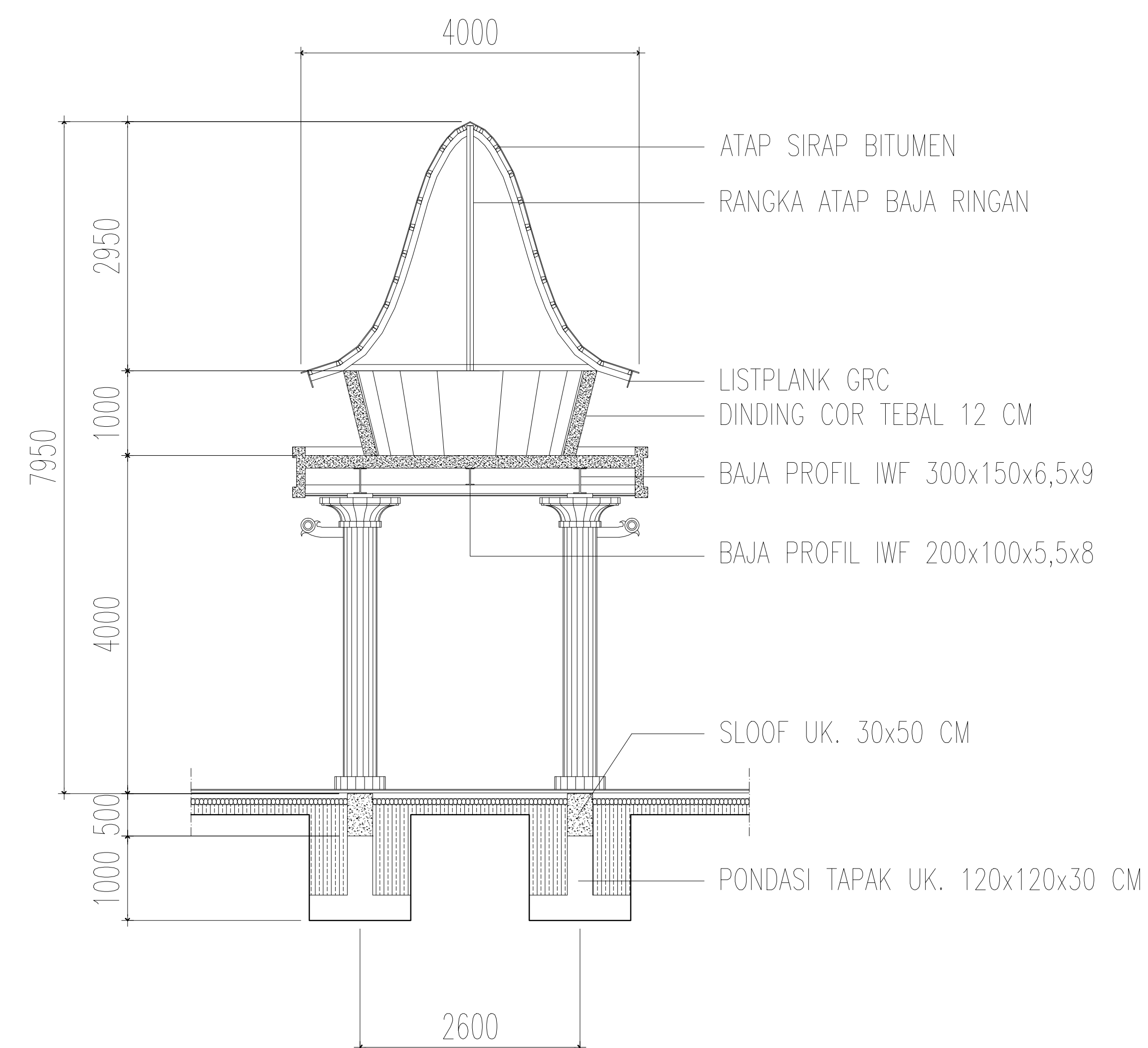
POTONGAN MEMANJANG GAPURA SKALA 1:100
