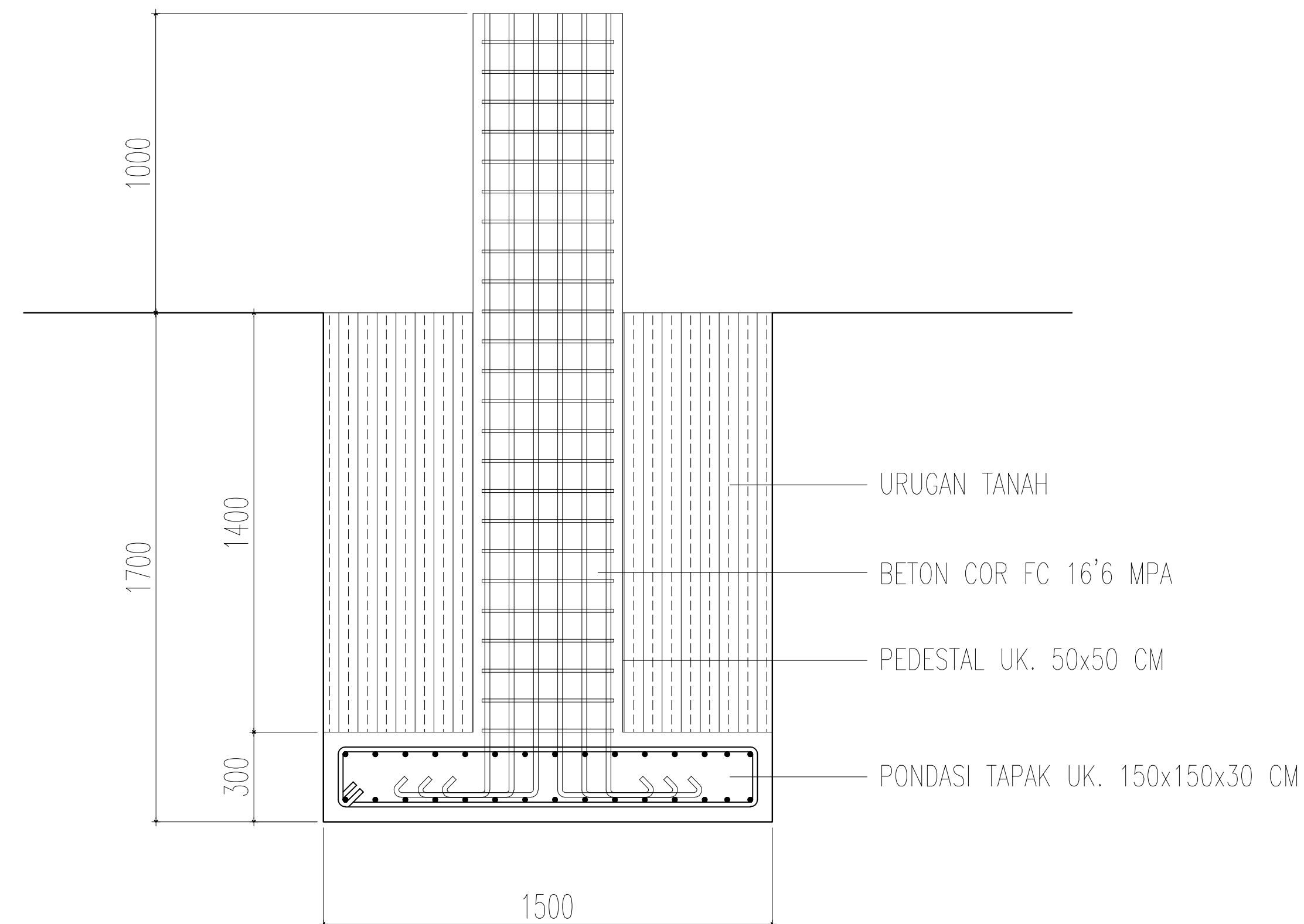
POTONGAN PONDASI TIANG BENDERA SKALA 1:100
