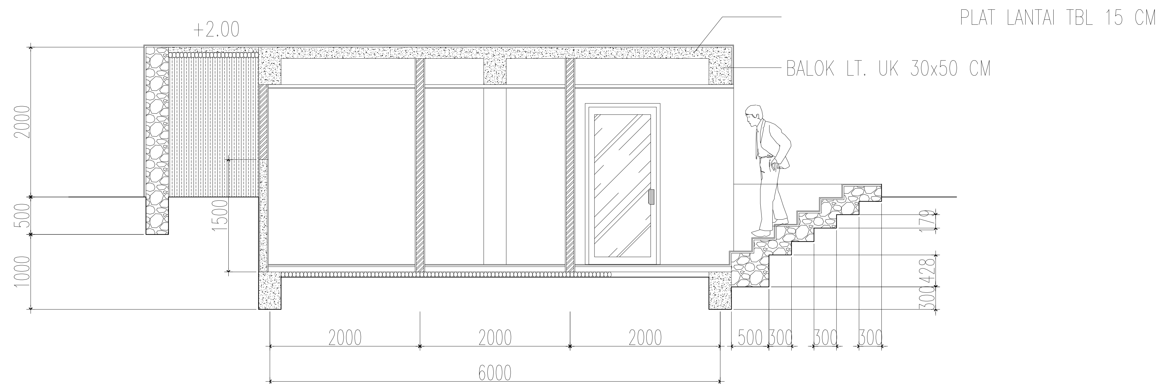
POTONGAN MELINTANG I SKALA 1:100
