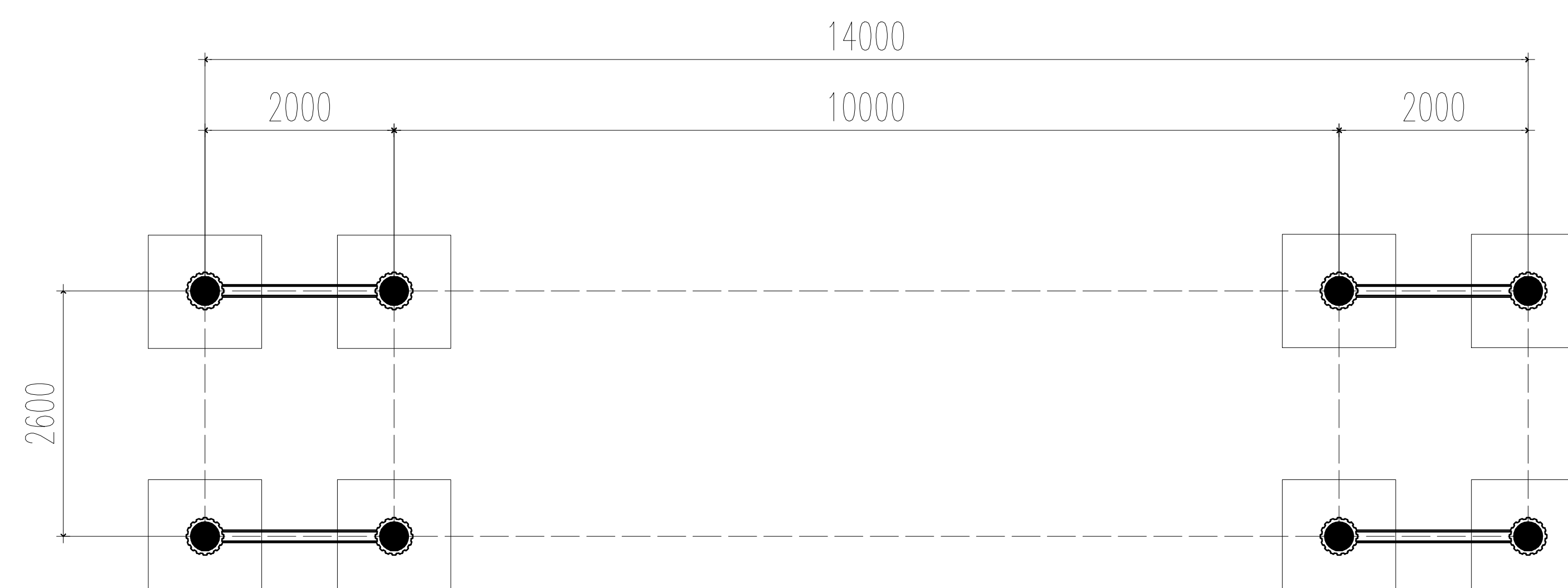
DENAH PONDASI TAPAK SKALA 1:100
