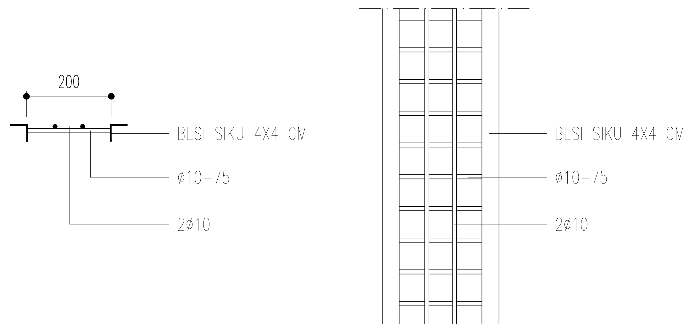
DETAIL GRILL PENUTUP PARIT SKALA : NTS
