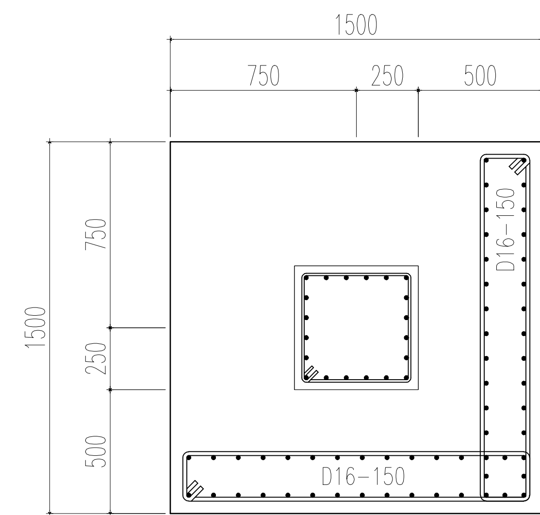
DENAH PONDASI TAPAK SKALA 1:100
