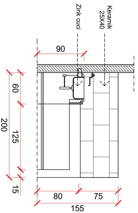
POTONGAN A-A SKALA 1:20
