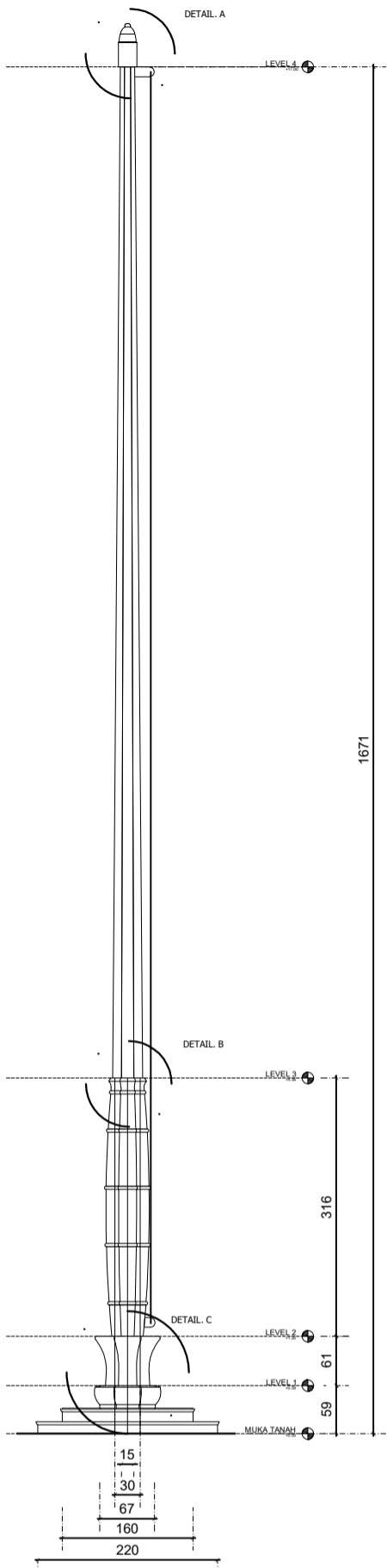
TAMPAK TIANG BENDERA (A) Skala 1 : 50
