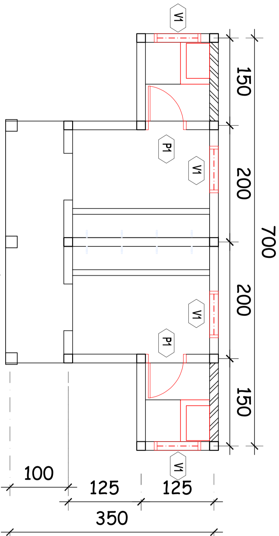
RENCANA KUSEN SKALA 1:50
