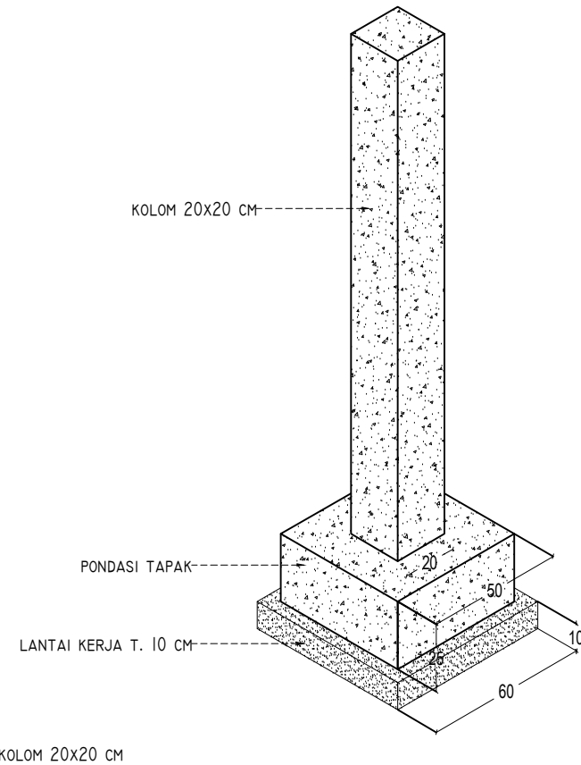
ISOMETRI PONDASI TAPAK SELASAR
