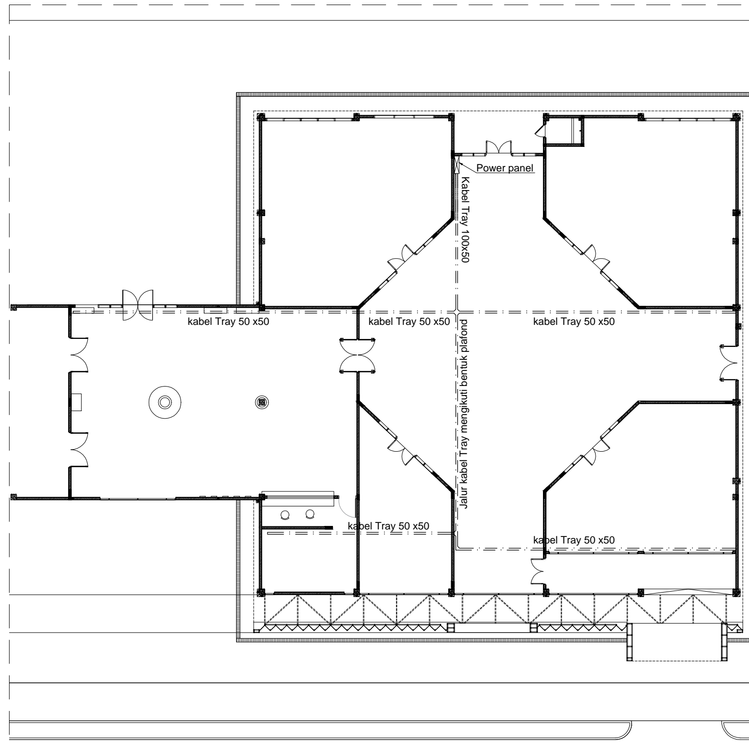
EL - INSTALASI TITIK STOP KONTAK SKALA 1:200
