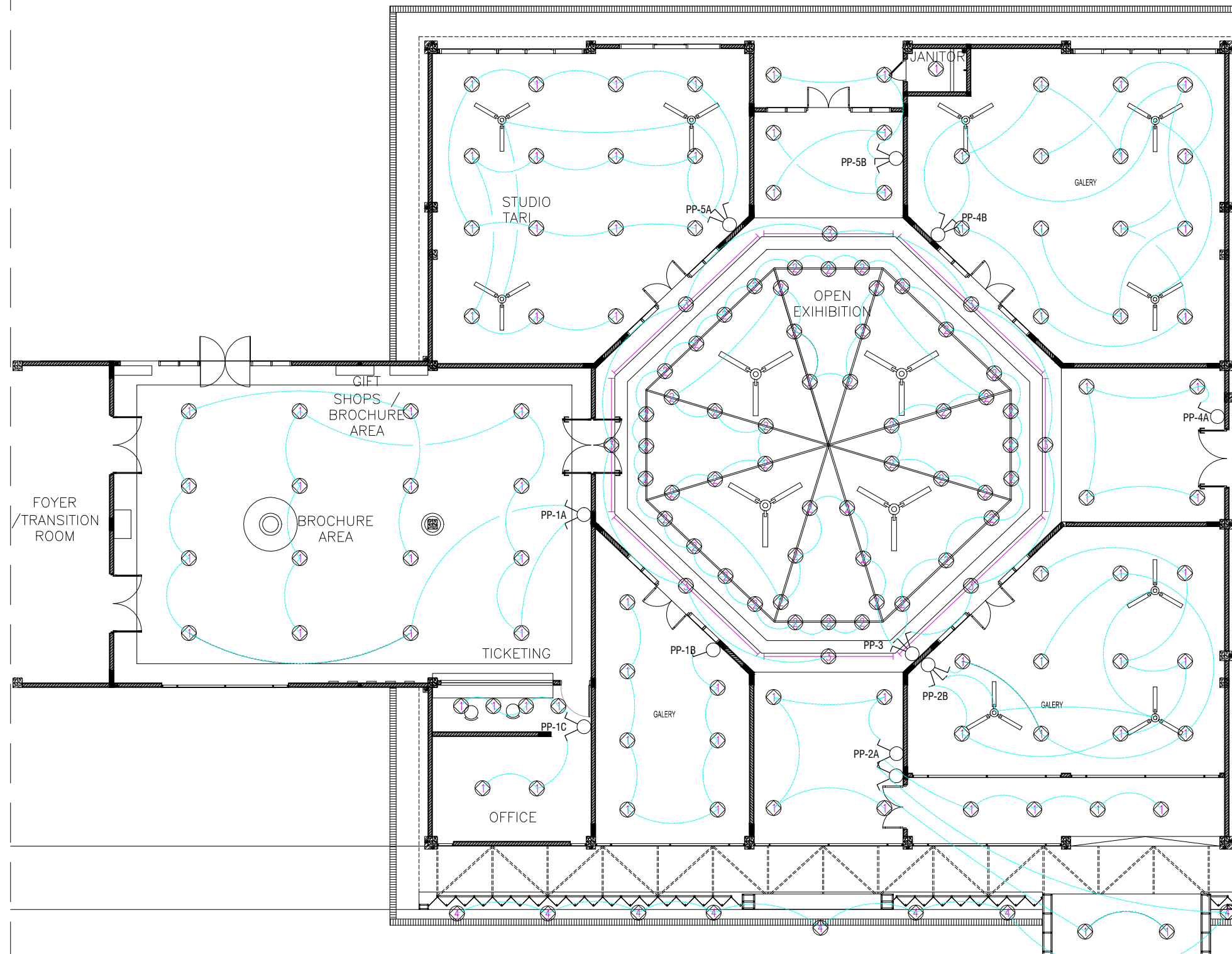
MEP INSTALASI TITIK LAMPU SKALA 1:150
