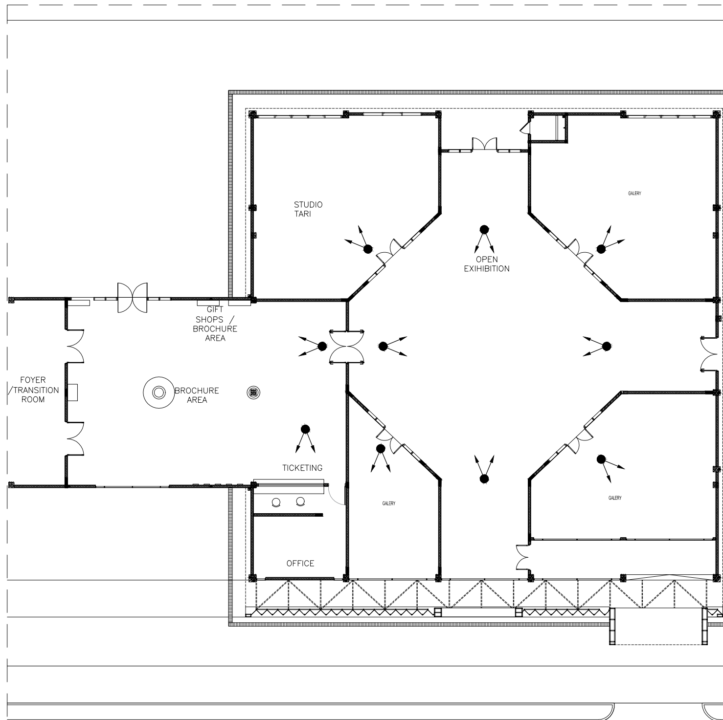
EL - INSTALASI TITIK OUTLET CCTV SKALA 1:200
