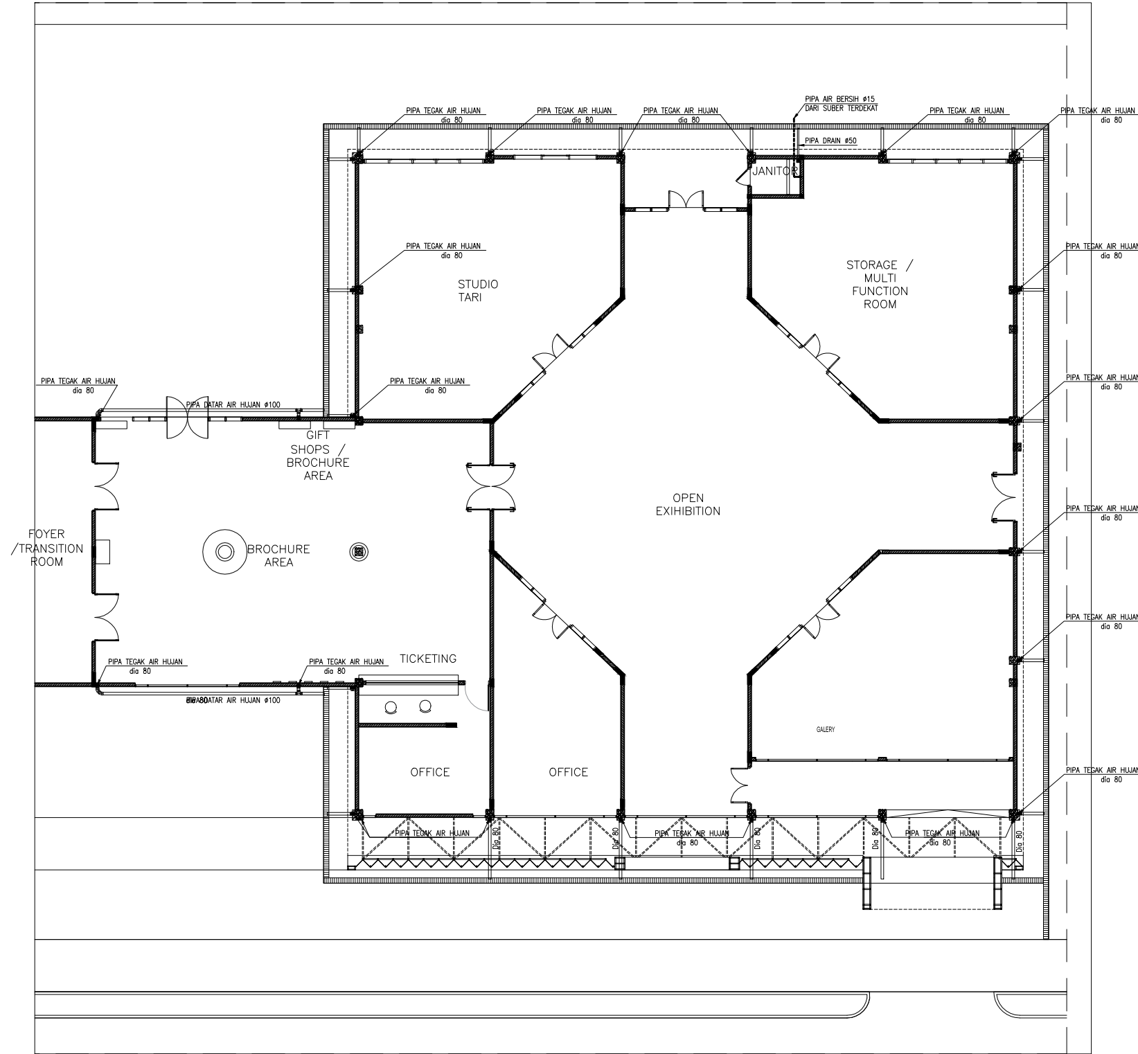
A1 INSTALASI PIPA AIR HUJAN LANTAI DASAR SKALA 1:200
