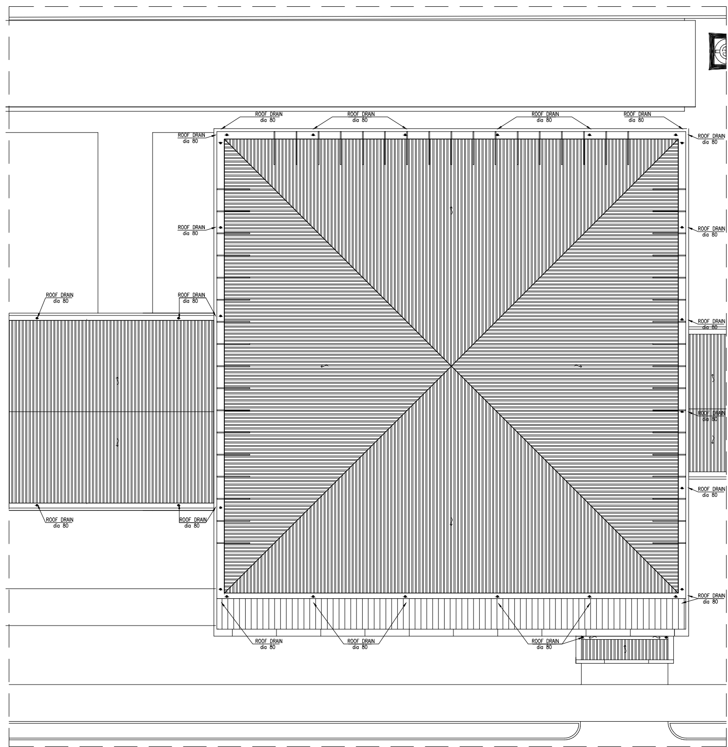
A1 - INSTALASI PIPA AIR HUJAN LANTAI ATAP SKALA 1:200
