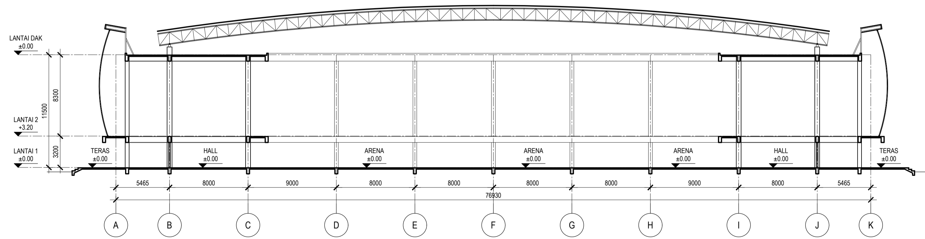
A POTONGAN A 1:250
