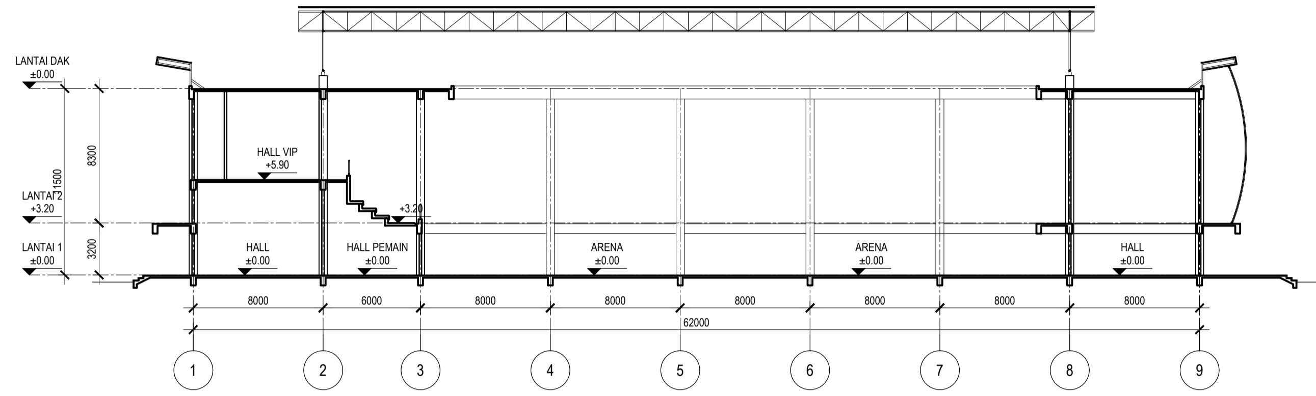
B POTONGAN B 1:250
